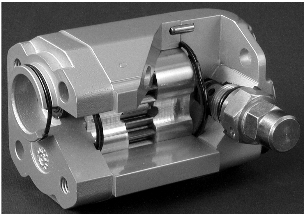
SNP1IN 03CA (カットアウェイ)
