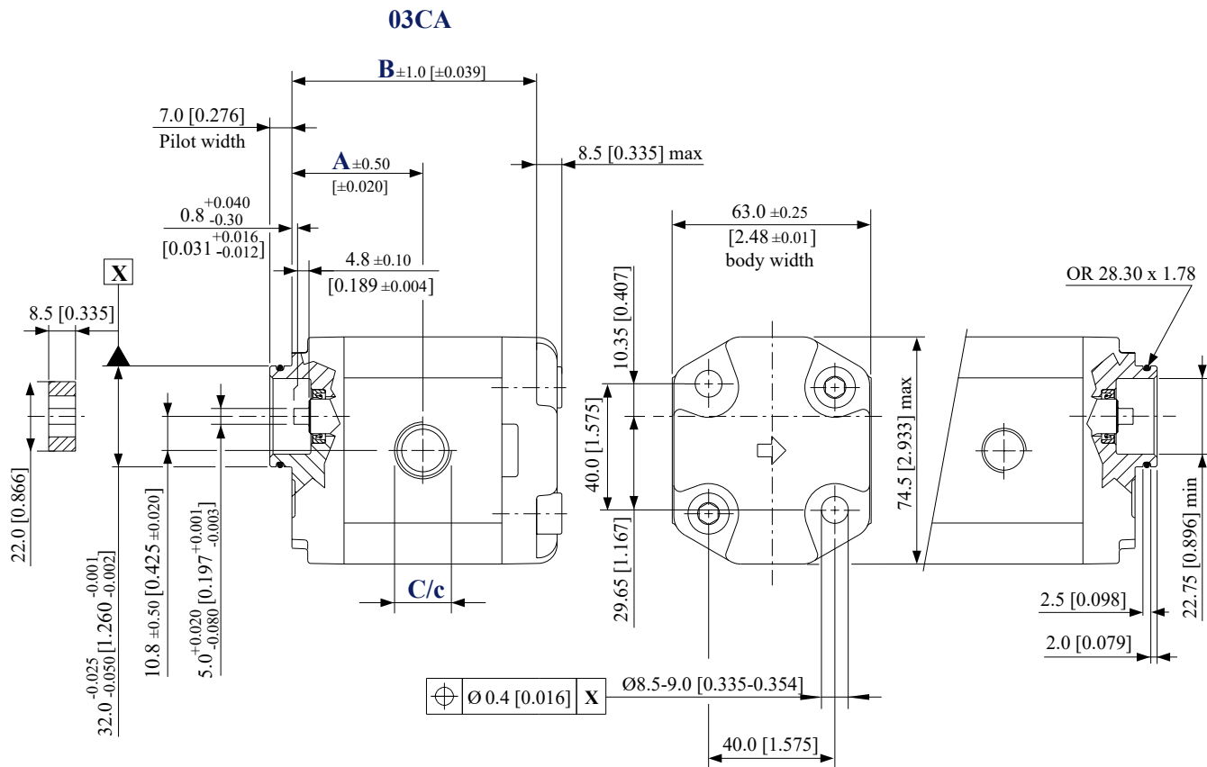
SNP1NN - 03CA 寸法
