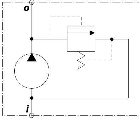
バルブ回路図
