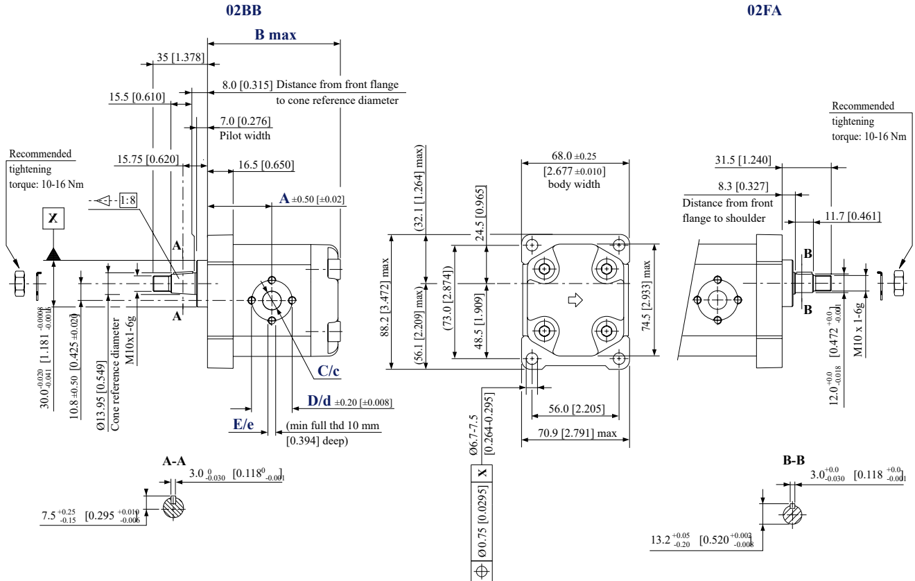
SKP1NN – 02BB および 02FA 寸法
