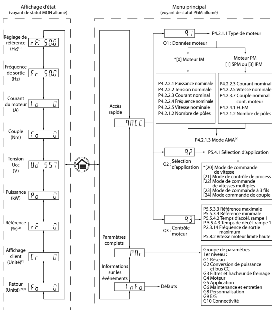
Illustration 2: Fonctionnement avec le panneau de commande
