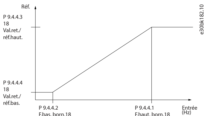
Illustration 84: Entrée impulsions
