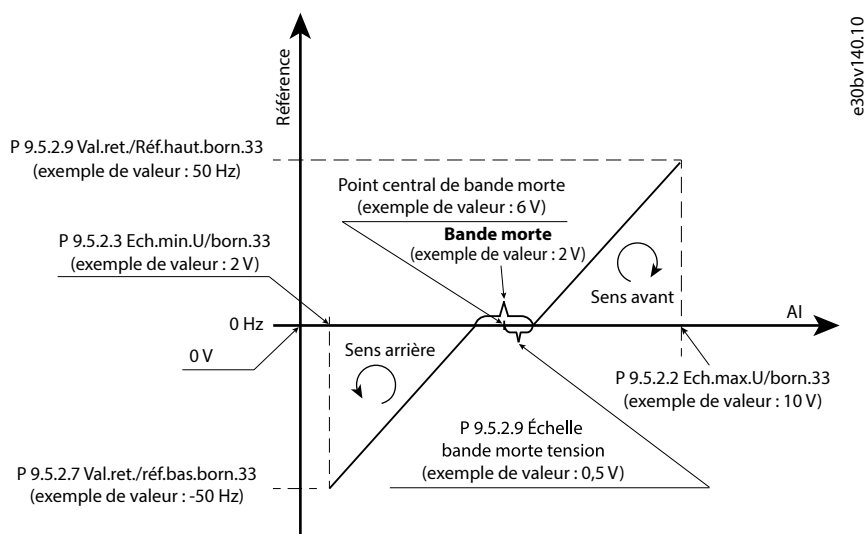
Illustration 86: Exemple de fonction de bande morte
