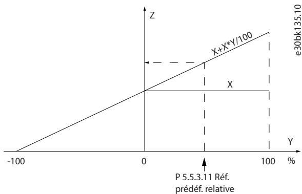
Illustration 76: Référence réelle
