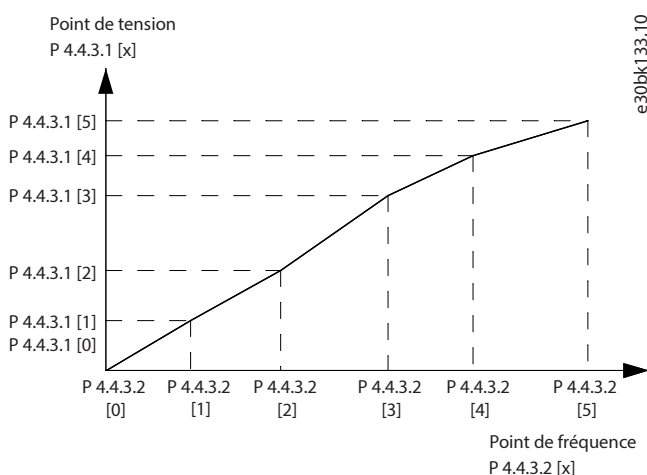
Illustration 70: Exemple de caractéristique U/f
