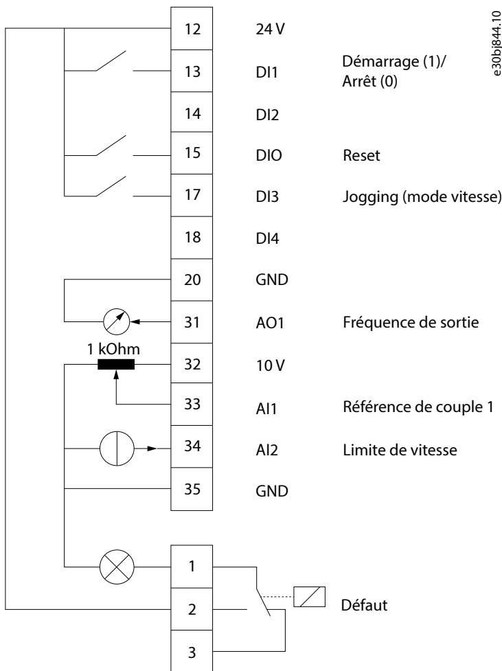
Illustration 42: Connexions par défaut
