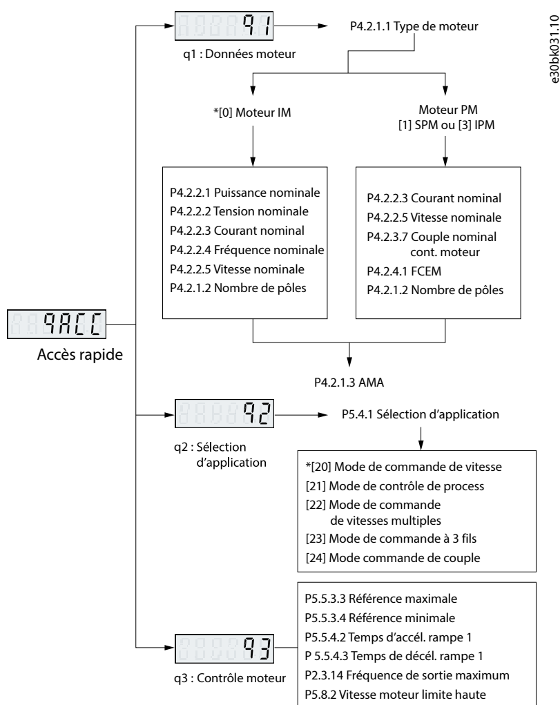
Illustration 5: Fonctions d'accès rapide
