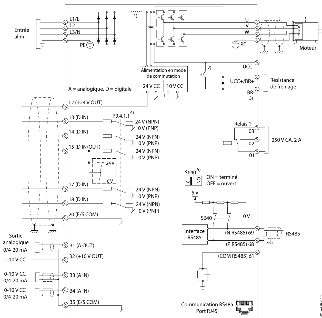
Illustration 35: Schéma de câblage
