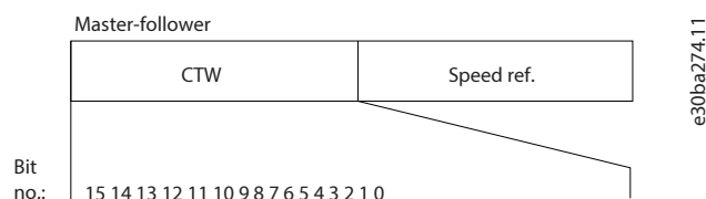
Illustration 65: Mot de contrôle selon le profil FC
