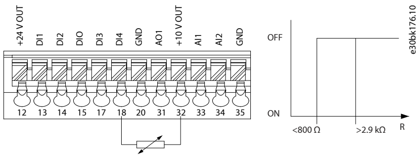
Illustration 73: Connexion de la thermistance PTC - entrée digitale
