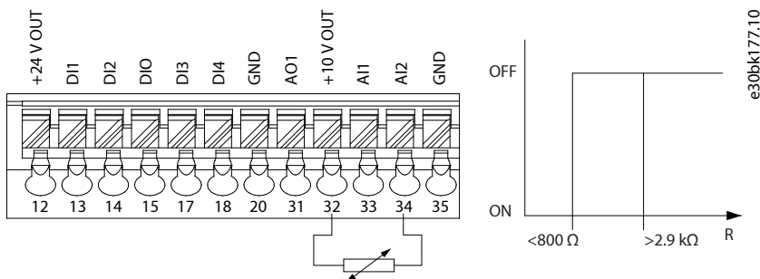
Illustration 74: Connexion de la thermistance PTC - entrée analogique
