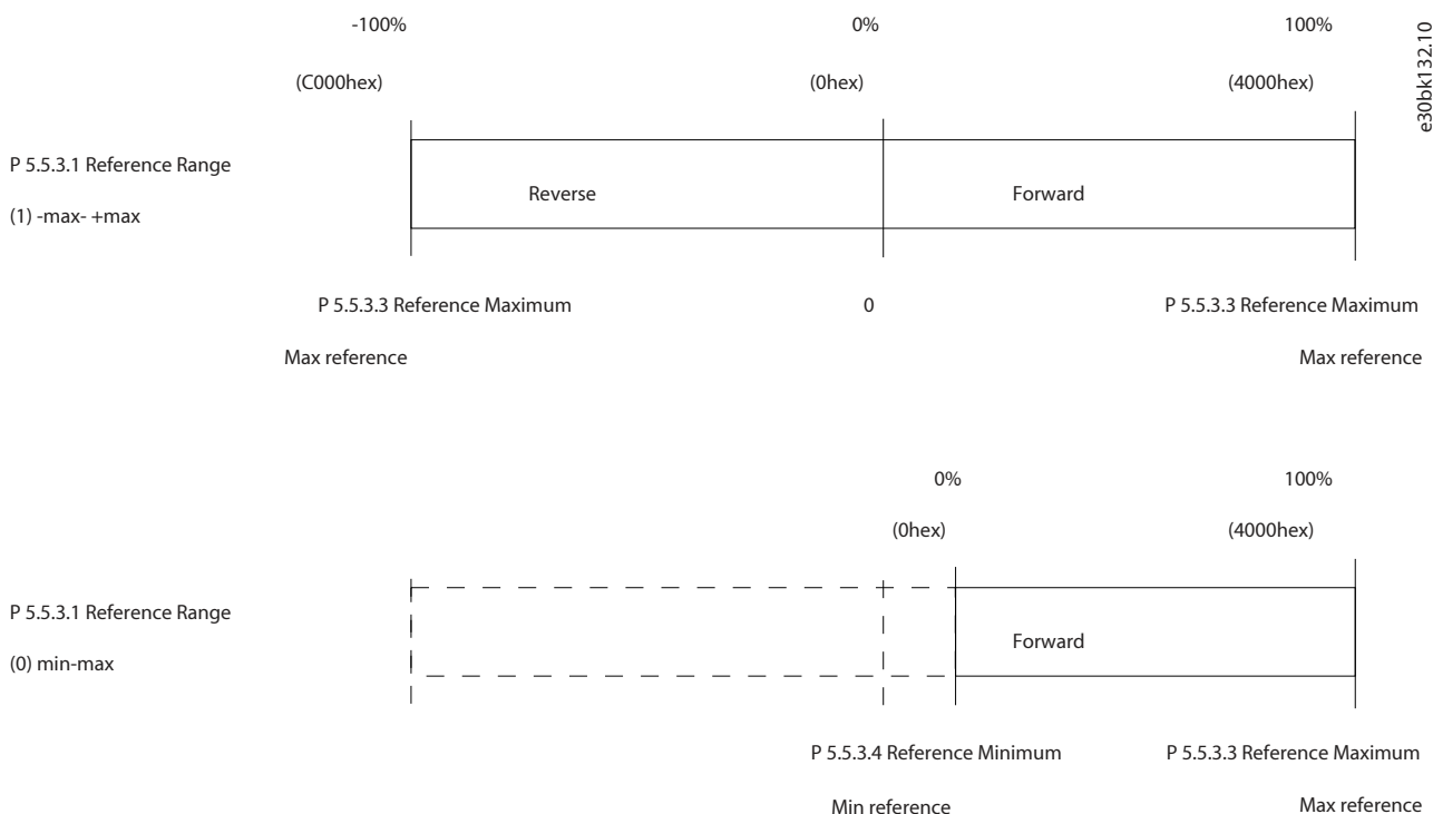
Illustration 68: Référence et MAV
