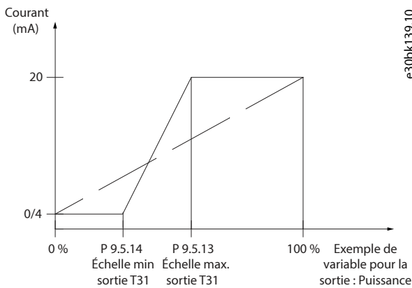
Illustration 85: Échelle de sortie en fonction du courant
