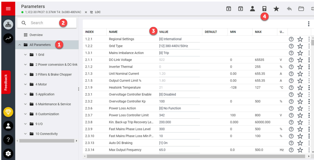
Illustration 22: Écran Paramètres
