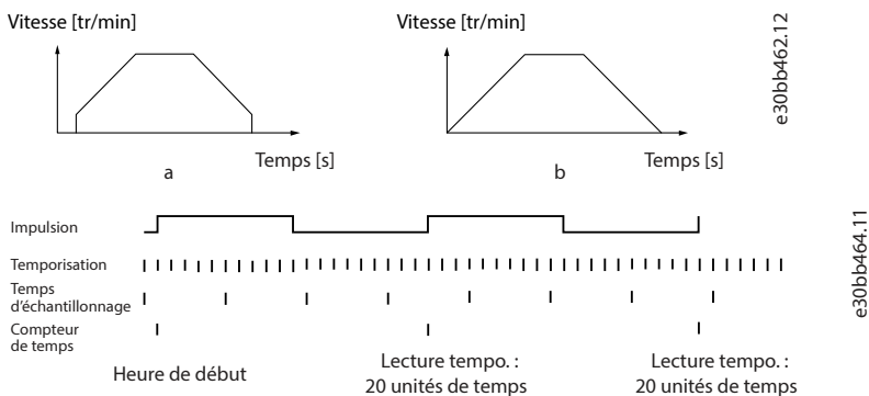
Illustration 81: Durée entre les flancs d'impulsion
