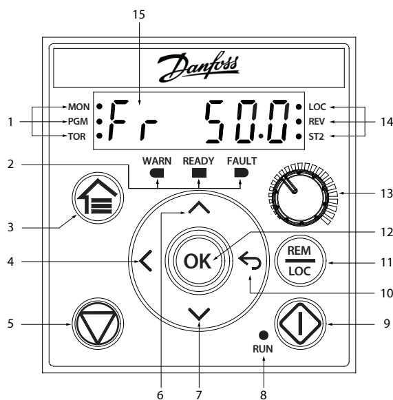
Illustration 1: Panneau de commande
