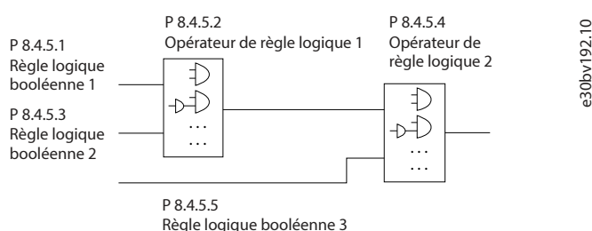
Illustration 80: Paramètres des règles logiques
