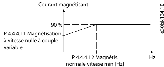
Illustration 71: Magnétisation du moteur
