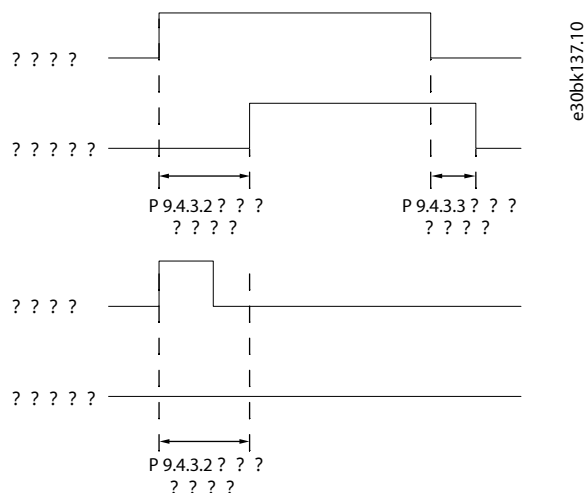
图 82: 继电器动作延迟
