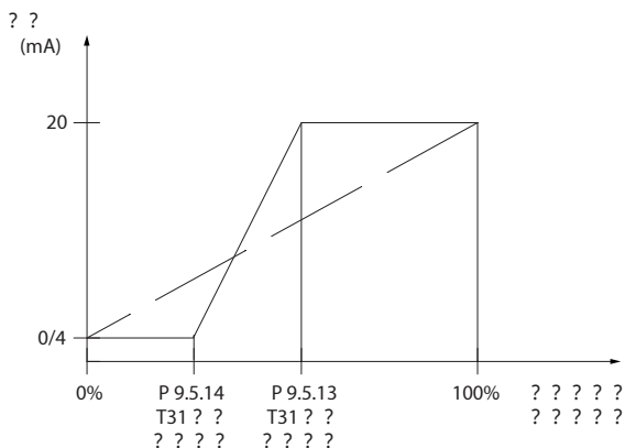
图 85: 输出对应电流标定
