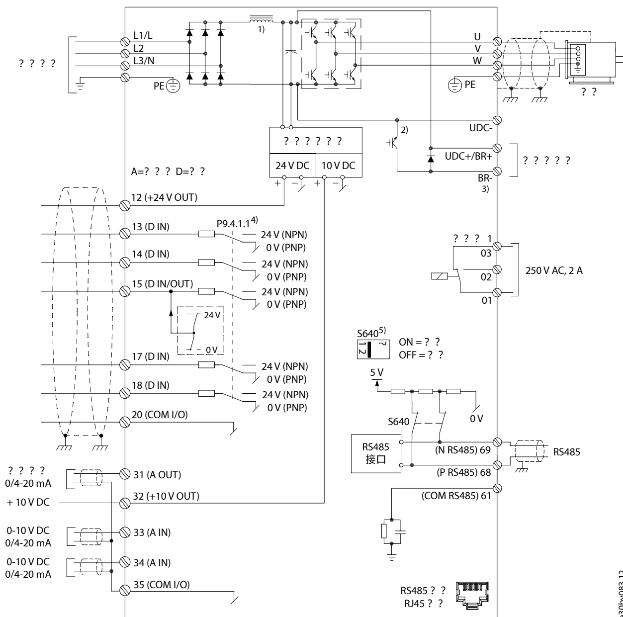
图 35: 接线图
