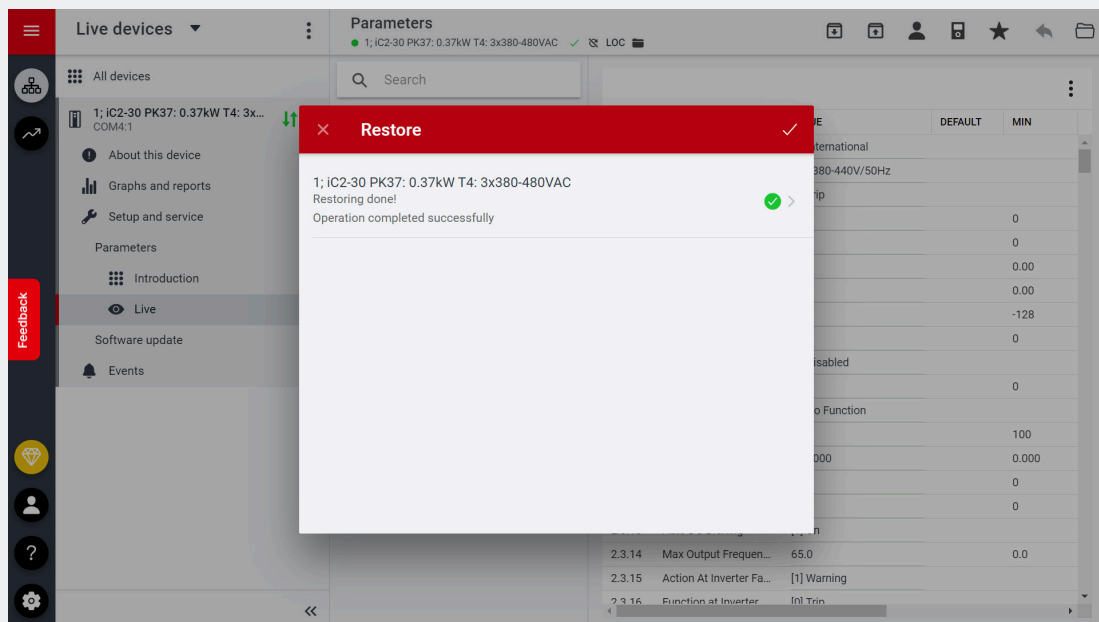
图 32: 恢复完成
