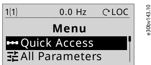
图 12: 菜单屏幕
