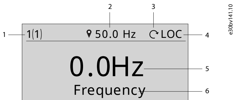
图 10: 主屏幕
