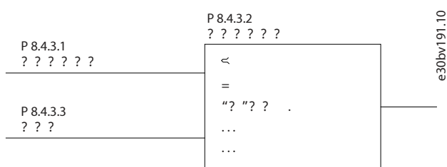
图 79: 比较器参数
