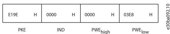
图 61: 报文
