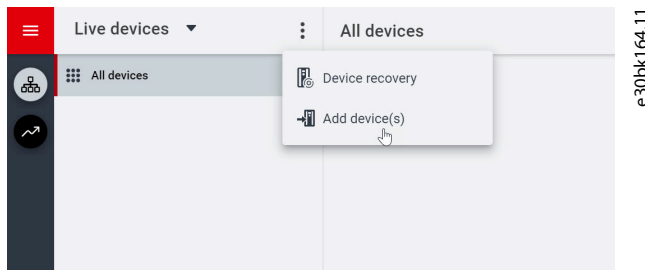
图 19: 建立连接
