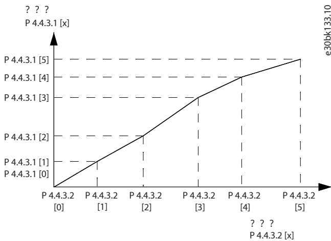
图 70: U/f 特性示例
