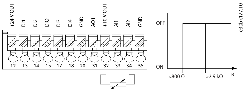
图 74: PTC 热敏电阻连接 - 模拟输入
