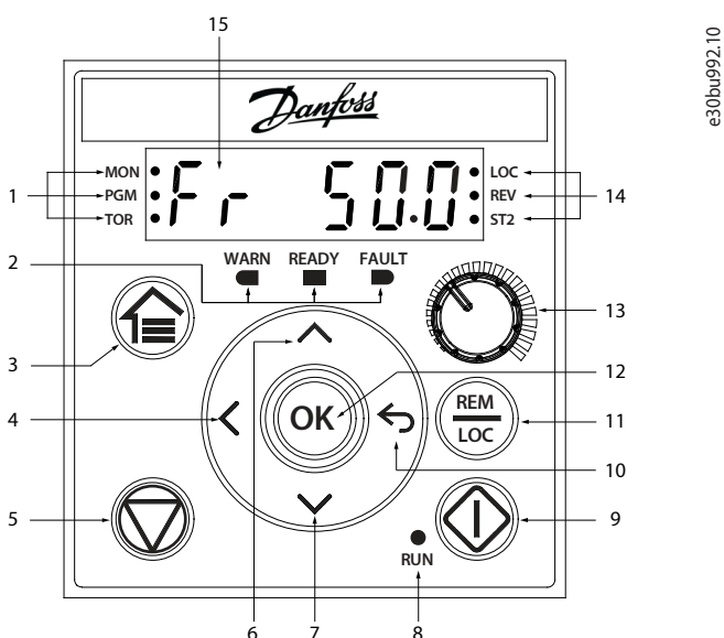
图 1: 控制面板
