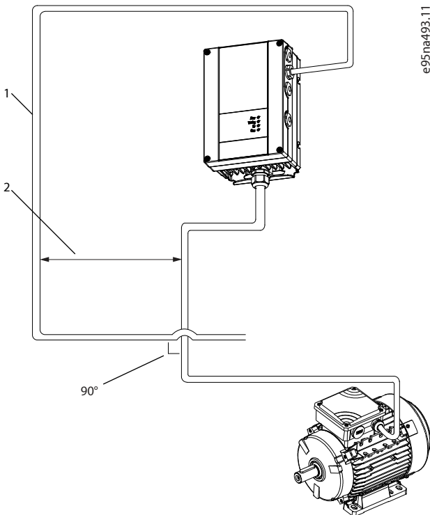
图 54: 通信电缆与电源电缆之间的最短距离
