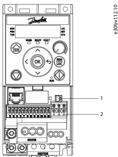
图 53: 终端电阻拨码开关的出厂设置
