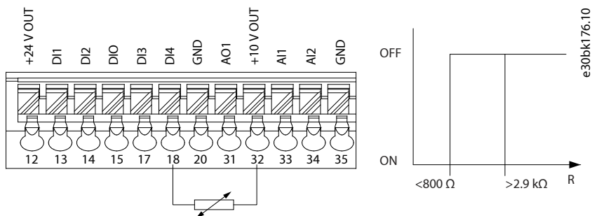
图 73: PTC 热敏电阻连接 - 数字输入
