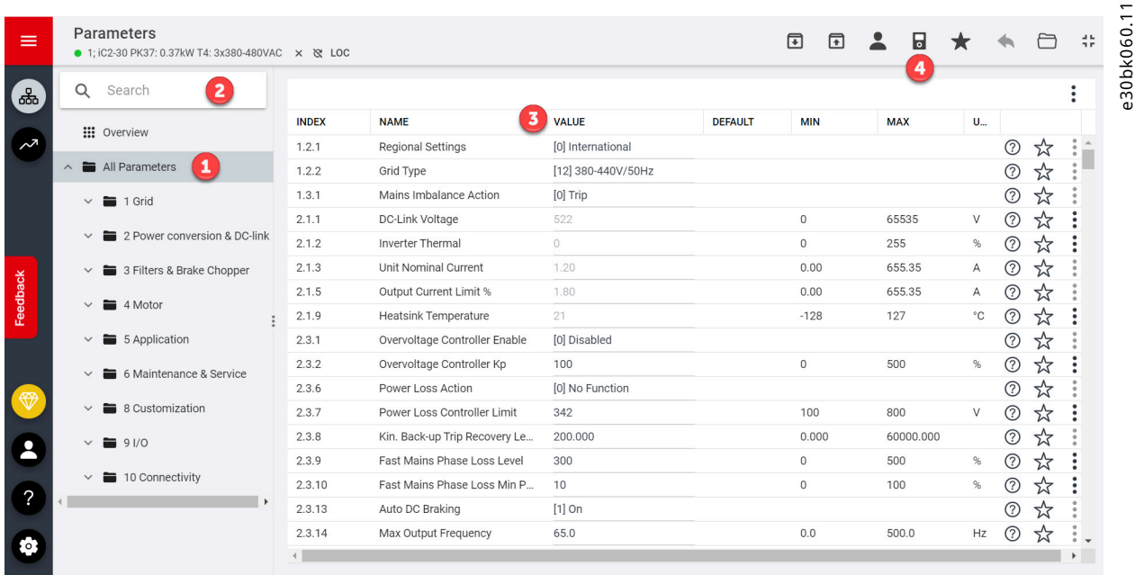
图 22: 参数屏幕
