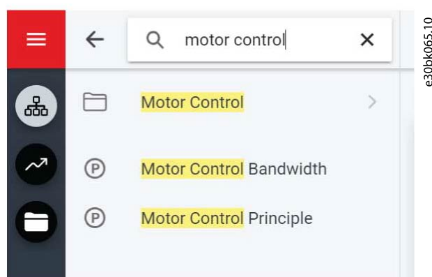
图 24: 搜索按钮
