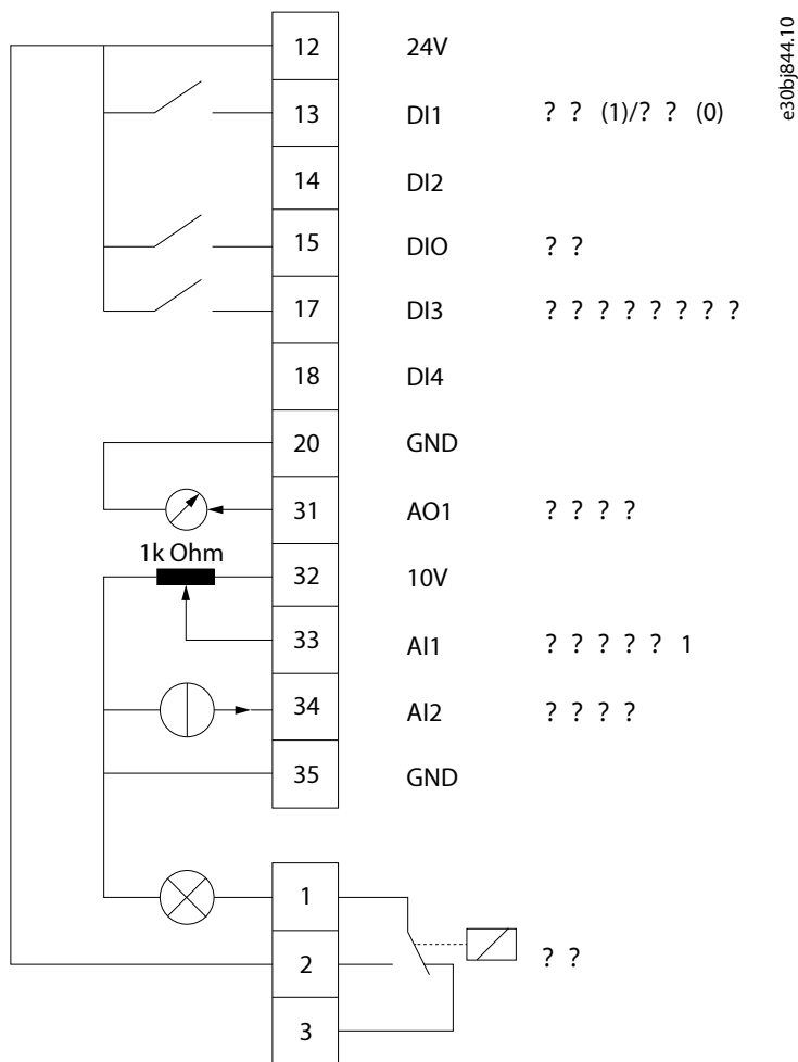
图 42: 默认连接
