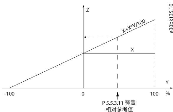
图 76: 实际参考值
