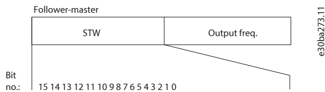
图 66: 状态字
