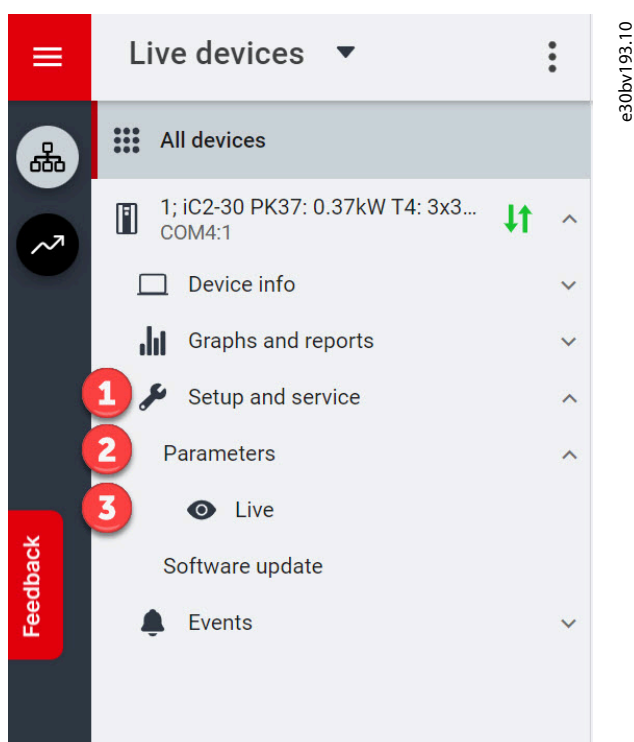
图 21: 设置和服务
