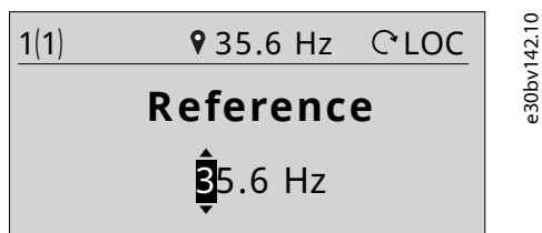
图 11: 设置参考值
