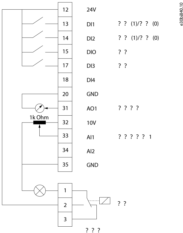
图 37: 默认连接
