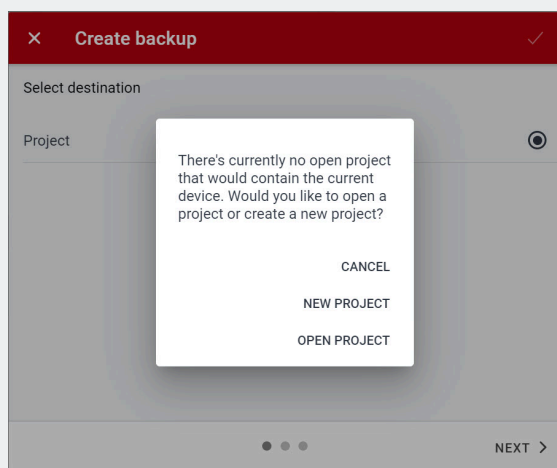
图 28: 备份目标
