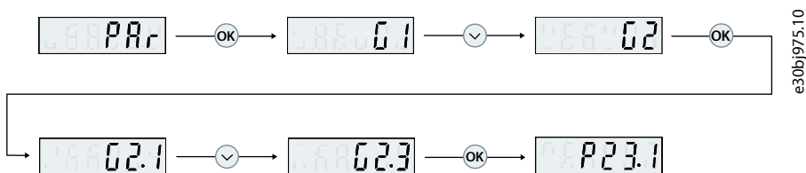
图 6: 参数导航
