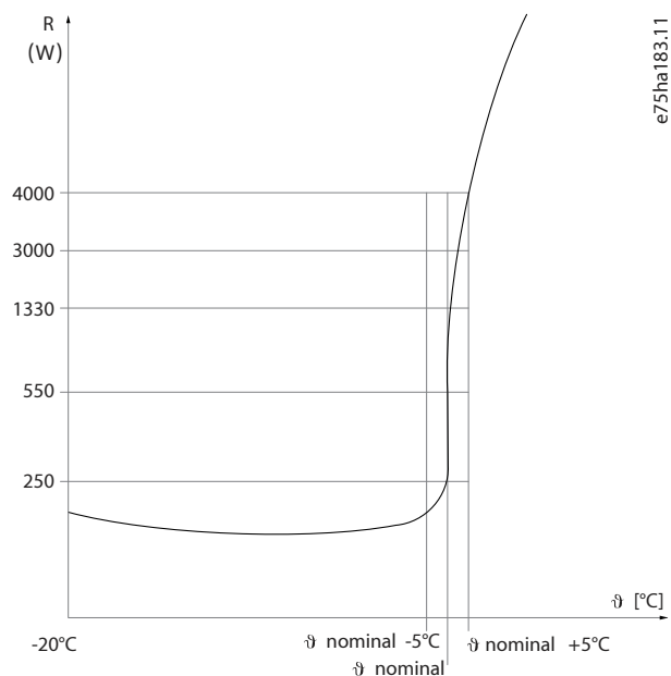
图 72: PTC 协议
