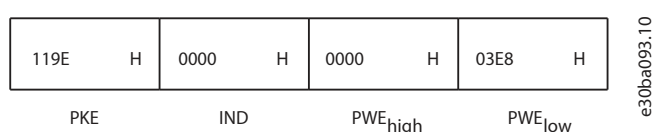
图 62: 主站响应
