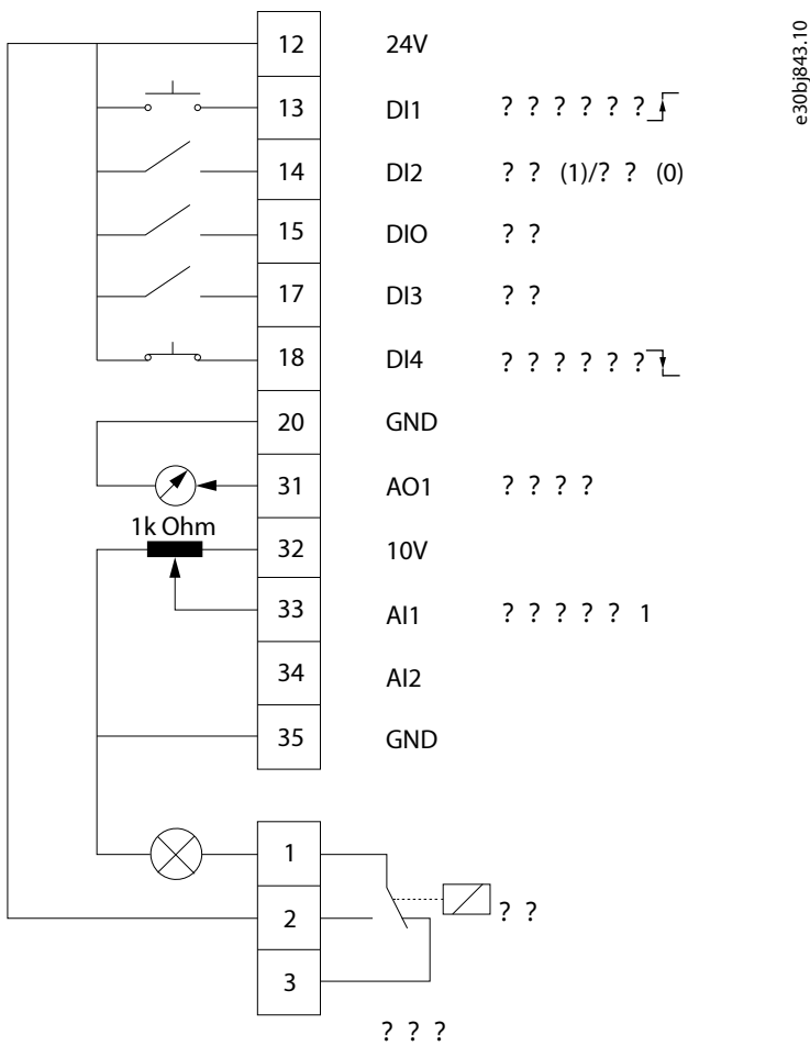
图 40: 默认连接
