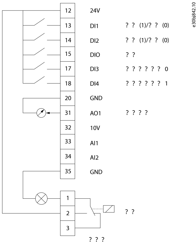
图 39: 默认连接
