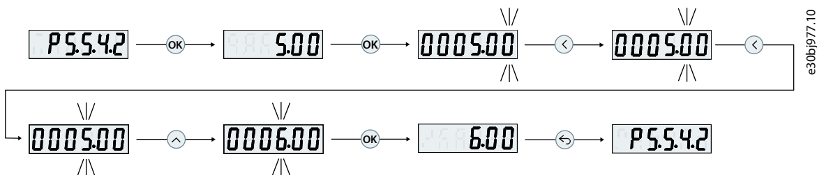
图 8: 更改参数值
