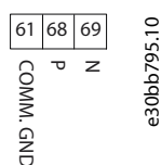
图 52: 网络连接
