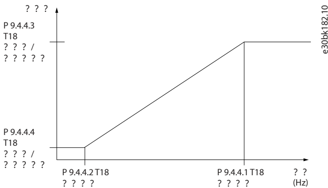
图 84: 脉冲输入
