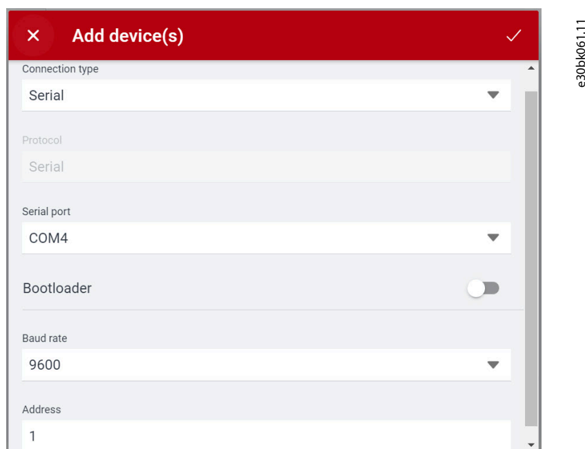
图 20: 串行连接
