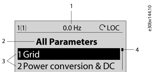
图 13: 参数组屏幕
