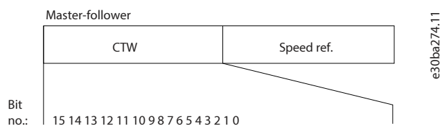
图 65: 与 FC 协议对应的控制字
