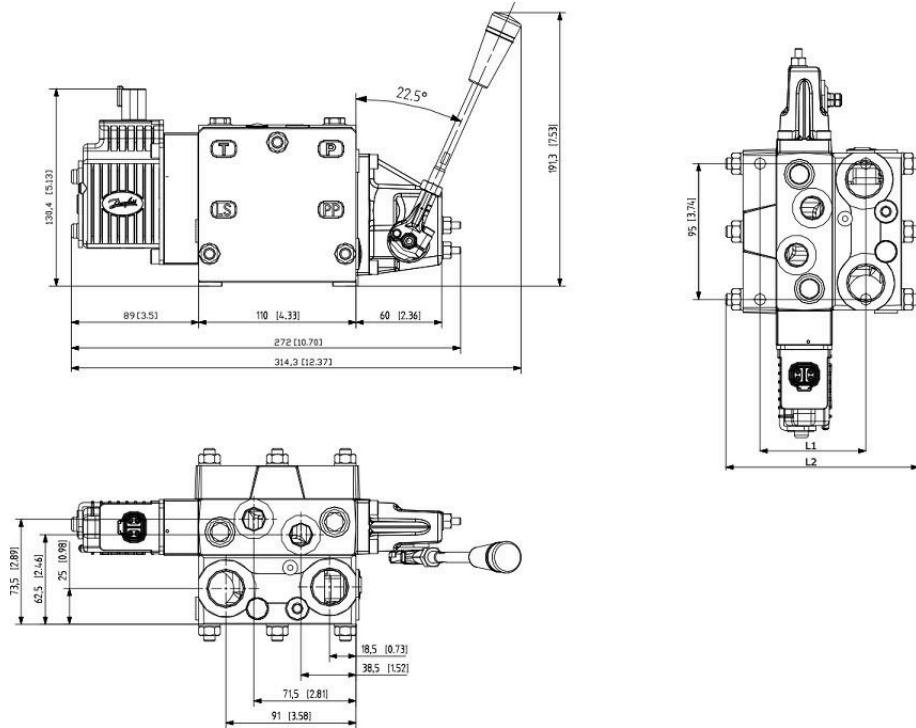
PVB 16 寸法 (12 セクション), mm [in]
