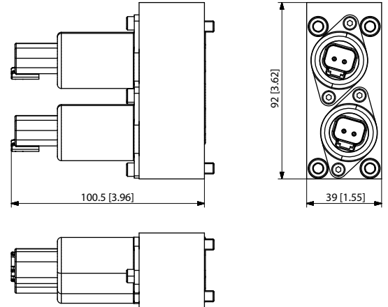
PVHC 寸法
