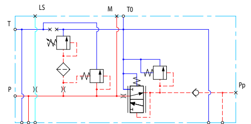
PPRV, T0 付クローズドセンタ PVP 回路図
