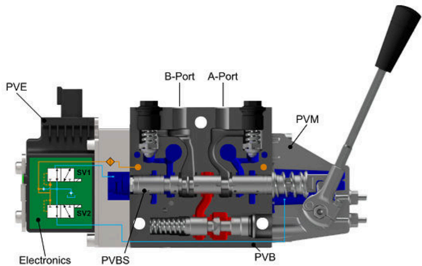
PVEO 付 PVG 16 断面図
