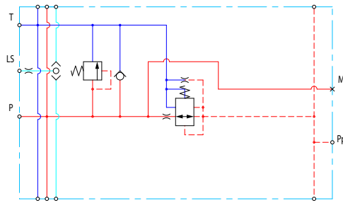
油圧回路図
