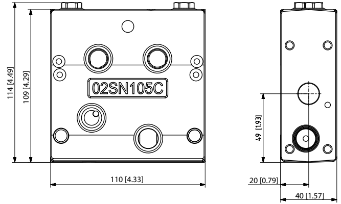
PVB 16 寸法
