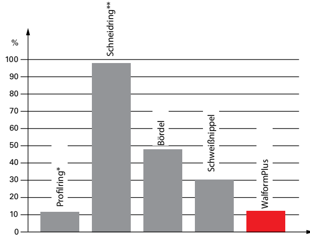
Vergleich der erforderlichen Montagewinkel
