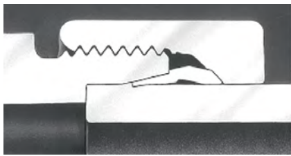
Schneidring – Deformation bei Überanzug
