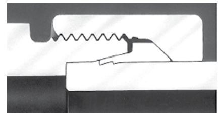
Profiling – Keine Deformation bei Überanzug
