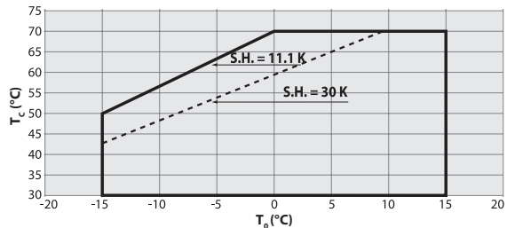
R134a - SZ084-185
