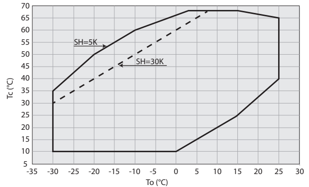
R410A - DSH240-600
