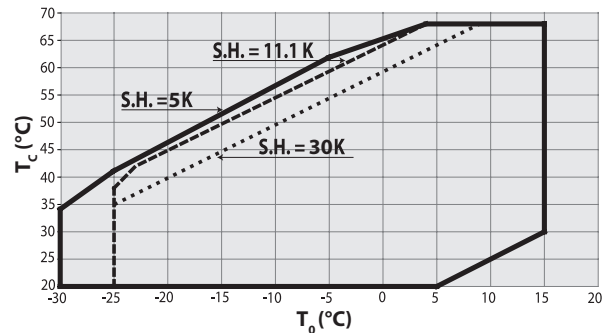
R410A - SH
