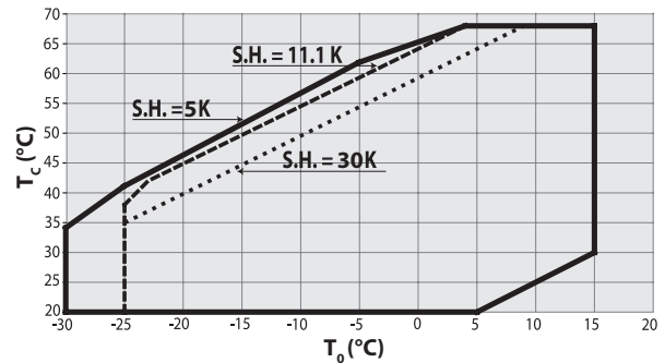
R410A - SH
