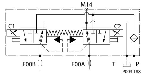
NFPE 回路図
