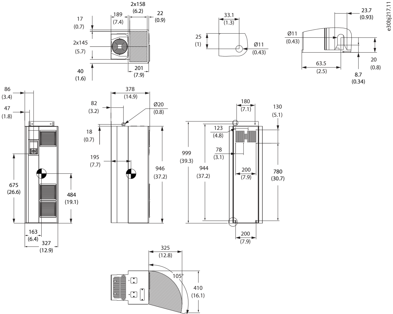
图 43: FB09a 尺寸
