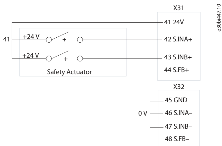
图 94: 使用相同极性的 STO 连接示例 (通道 A 和通道 B = 24 V)
