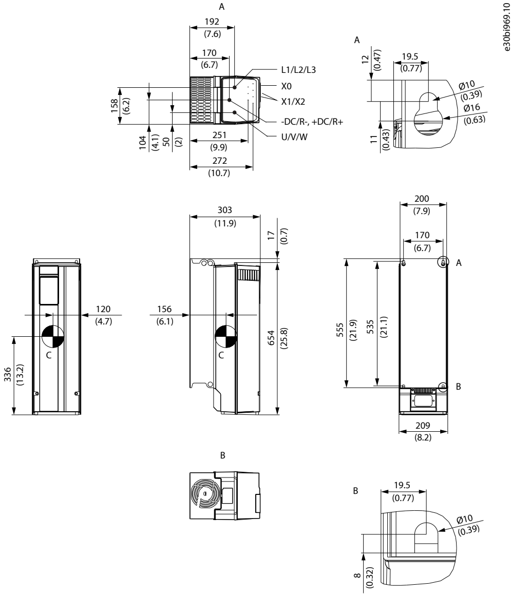
图 31: FK06 尺寸
