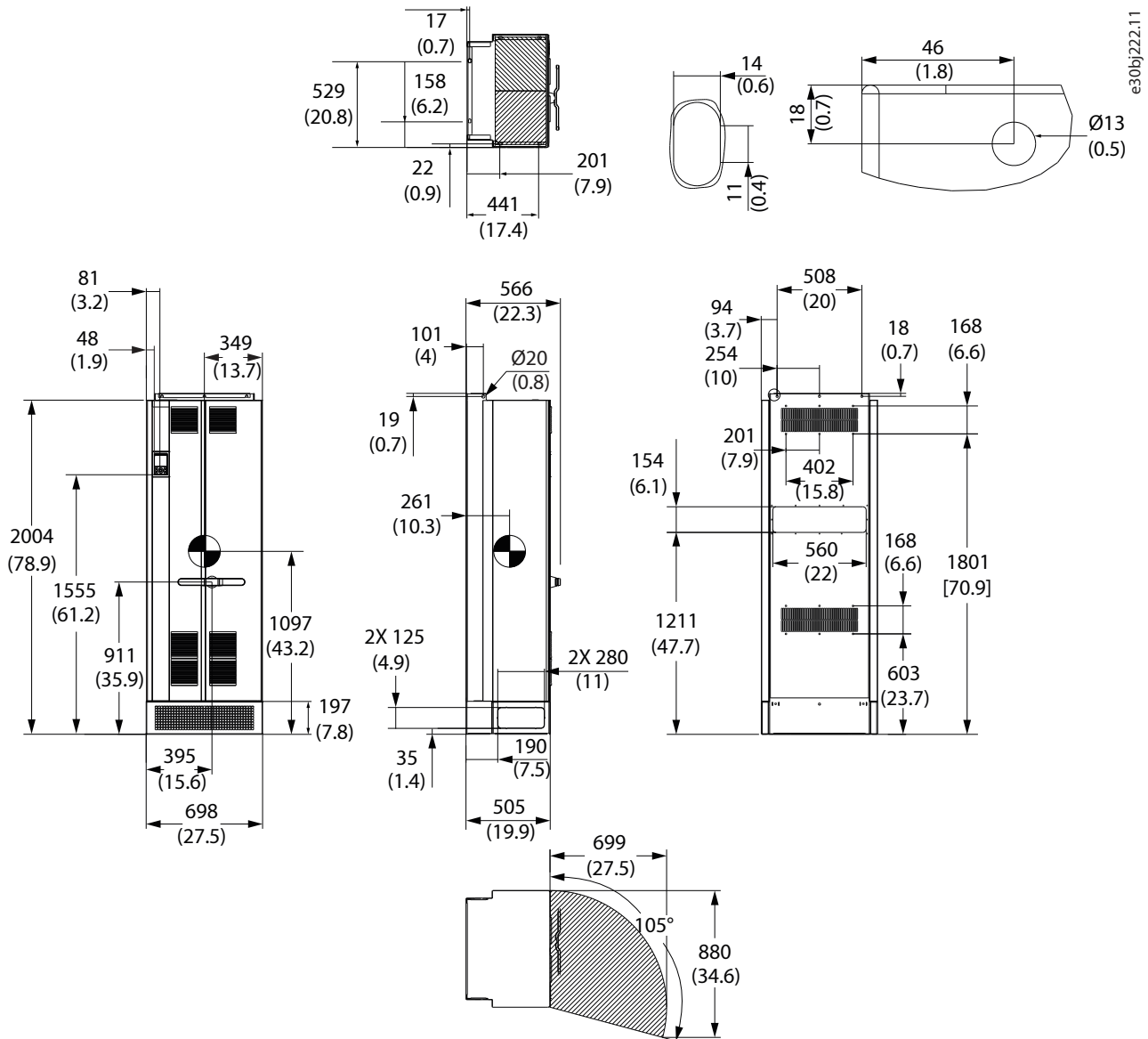
图 51: FB12 尺寸
