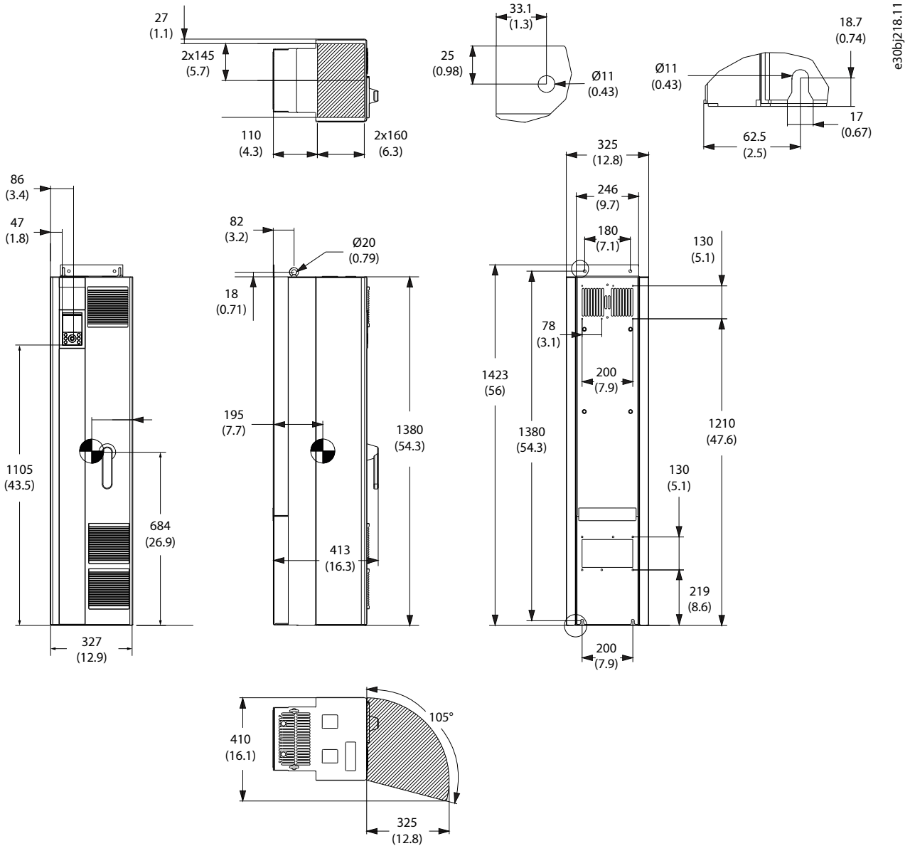
图 36: FK09c 尺寸
