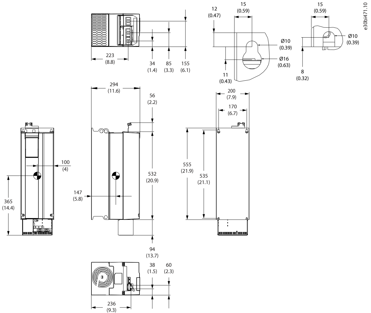
图 20: FA06 尺寸
