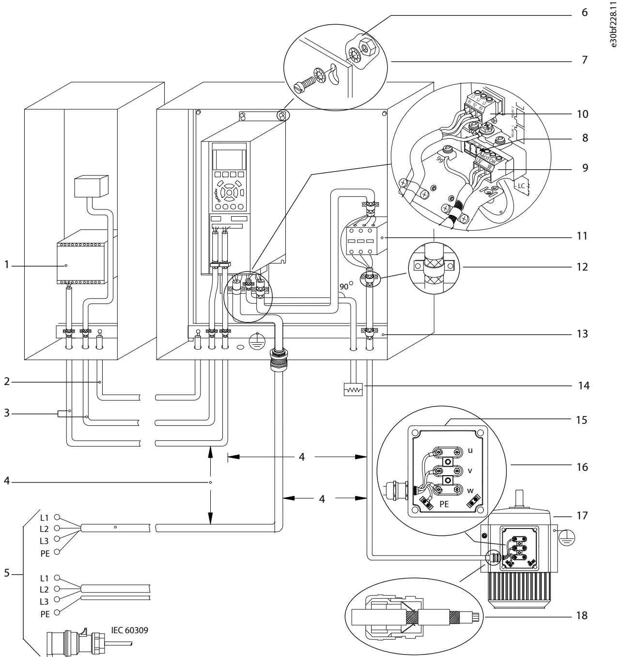
图 81: 正确的 EMC 合规安装示例
