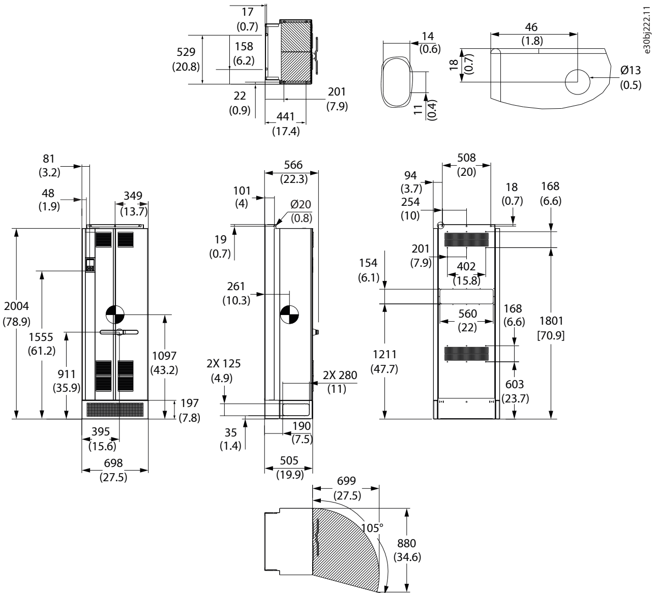
图 42: FK12 尺寸
