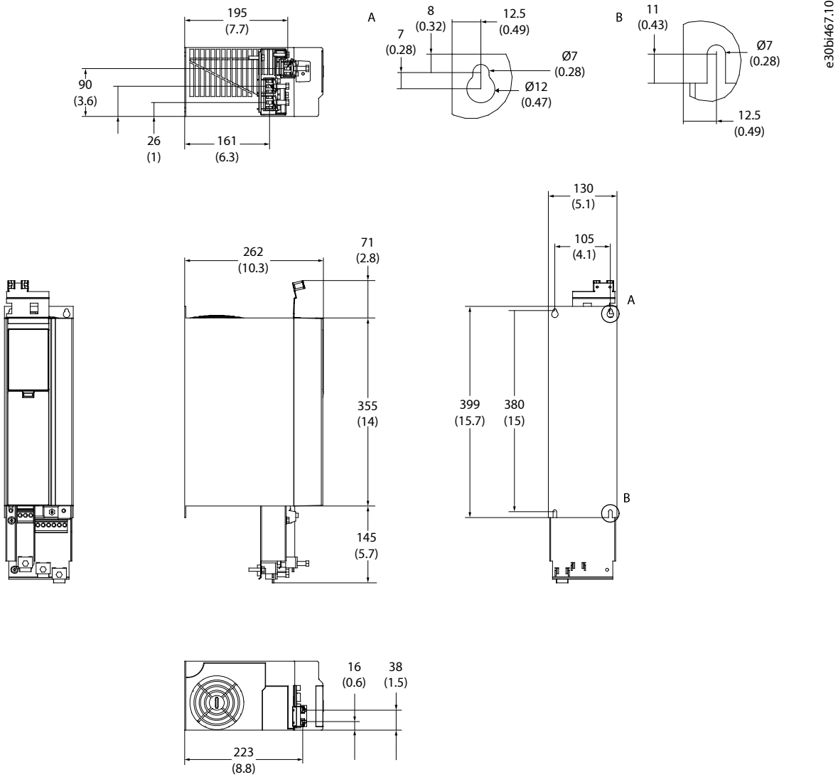
图 16: FA04a 尺寸
