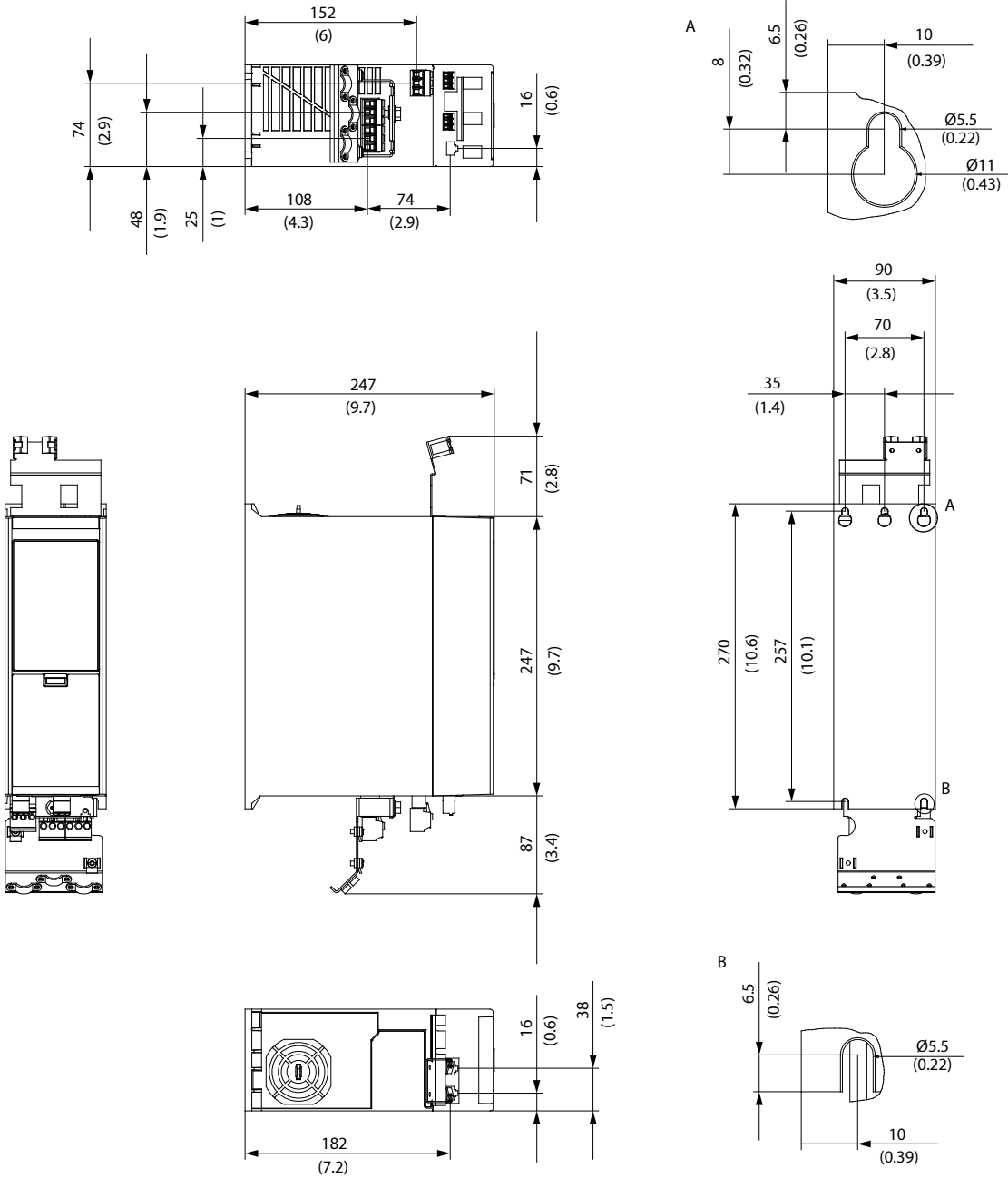
图 13: FA02b 尺寸
