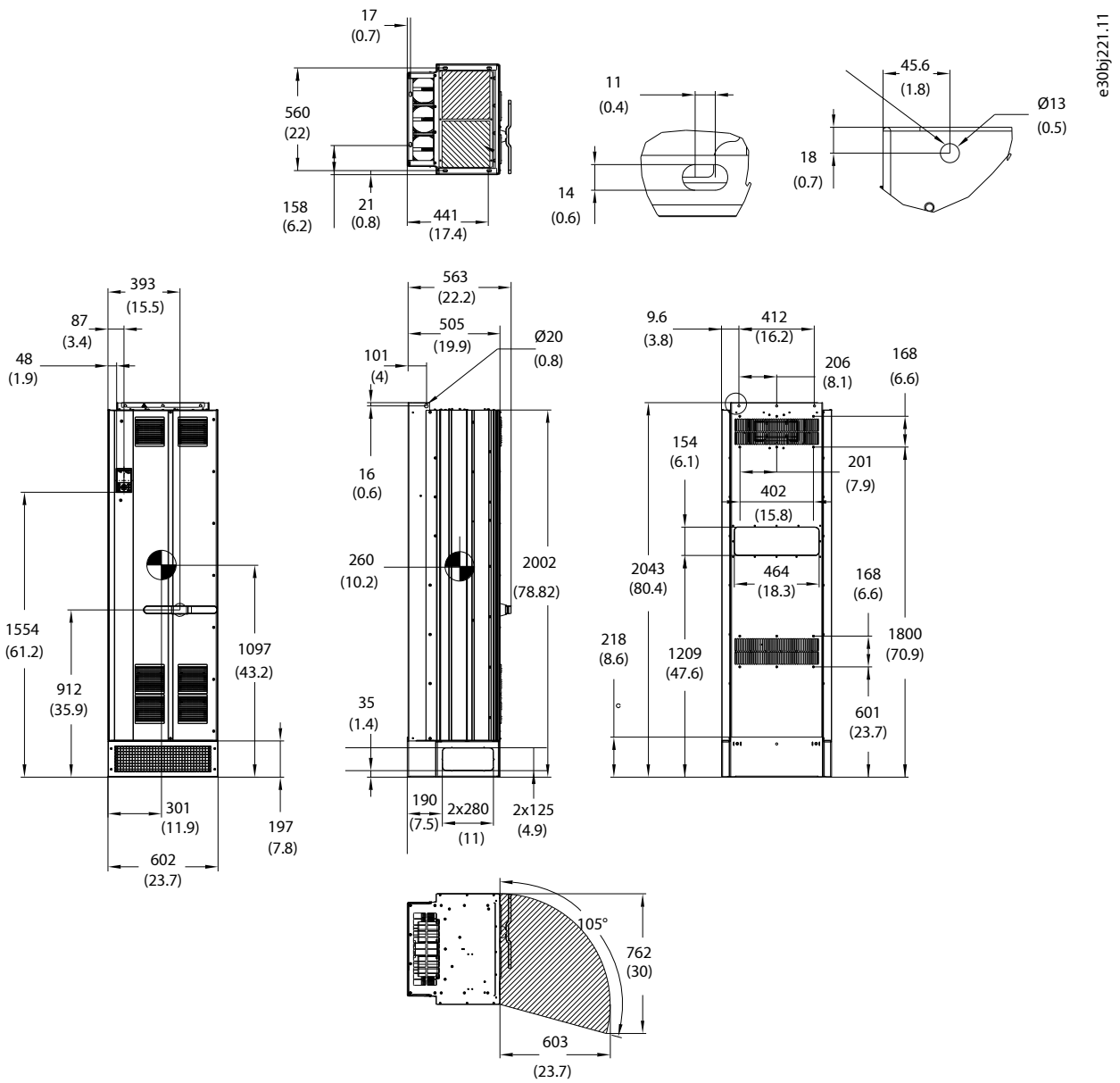
图 50: FB11 尺寸
