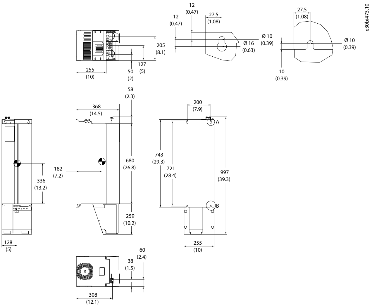
图 22: FA08 尺寸
