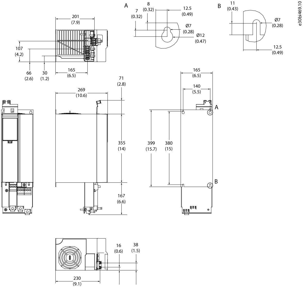
图 18: FA05a 尺寸
