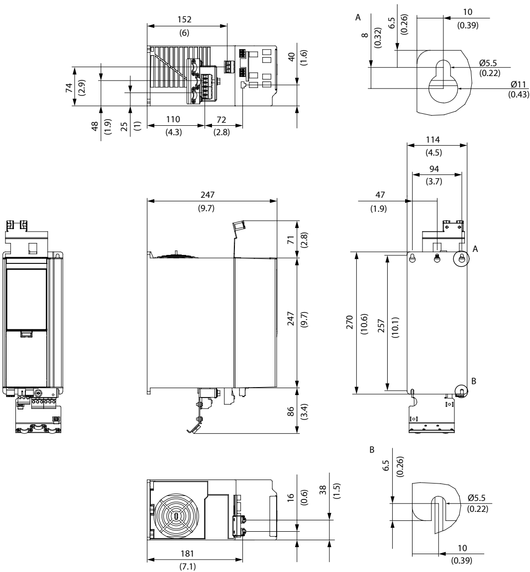
图 15: FA03b 尺寸
