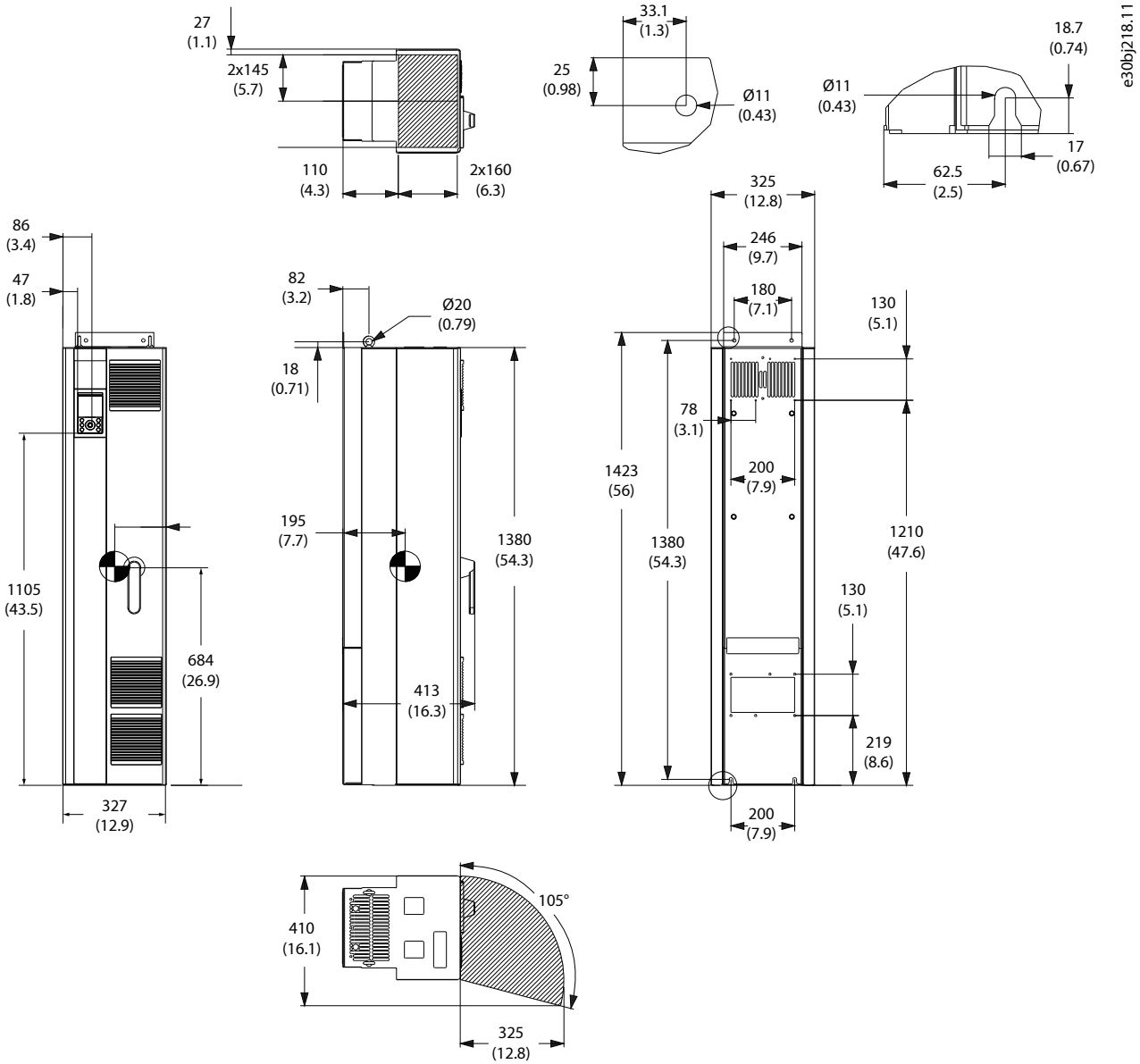
图 45: FB09c 尺寸
