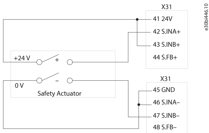
图 95: 使用不同极性的 STO 连接示例
