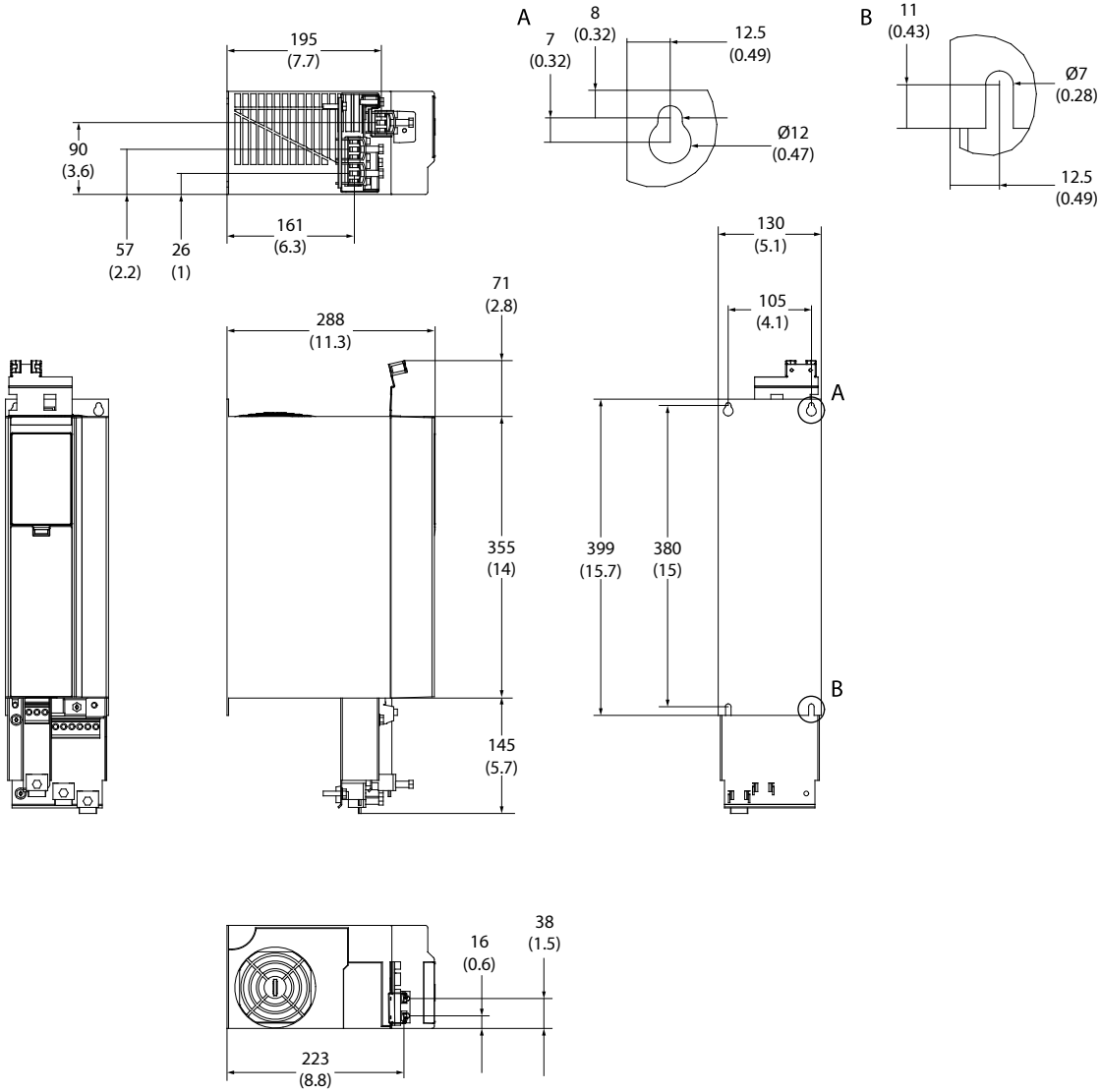
图 17: FA04b 尺寸
