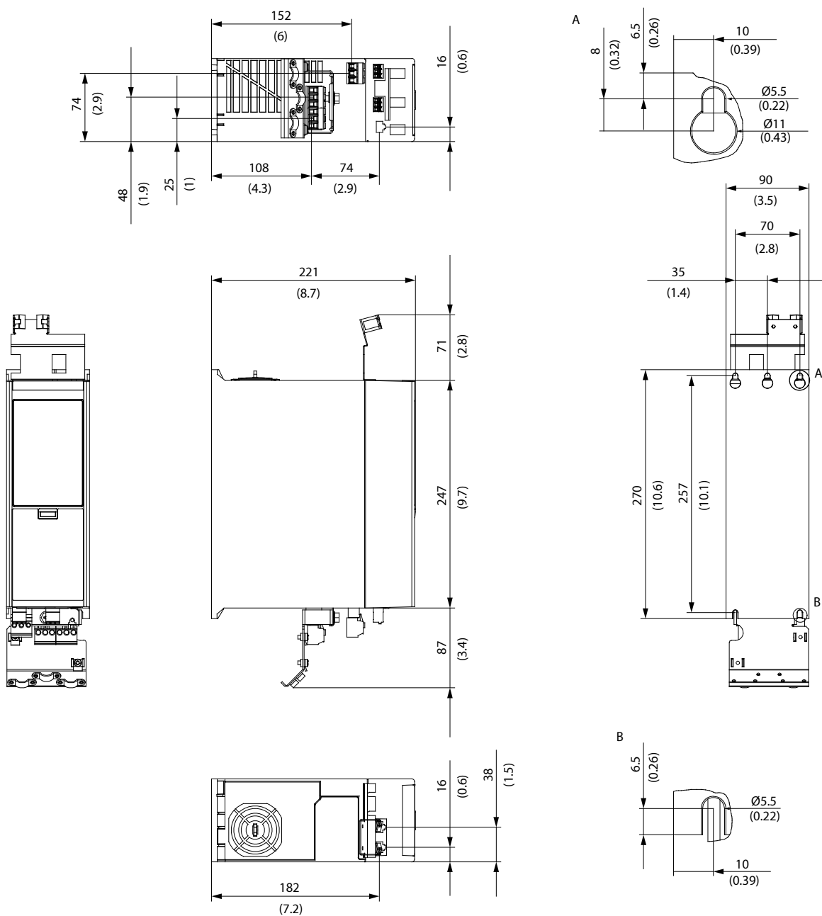
图 12: FA02a 尺寸
