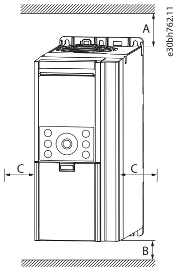
图 76: 冷却间隙
