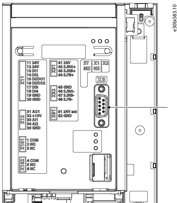
图 90: X8 连接器的位置
