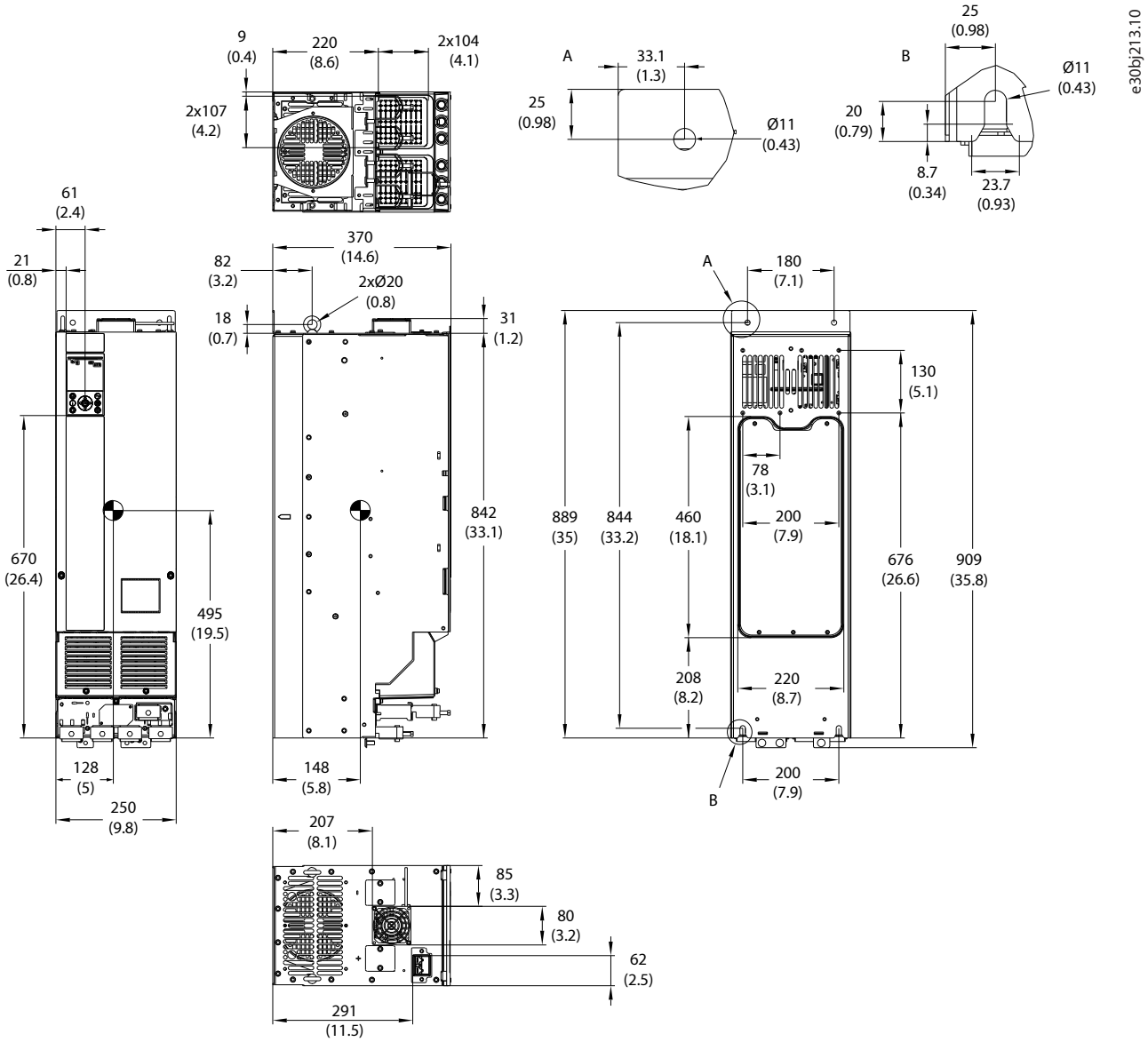
图 23: FA09 外部尺寸
