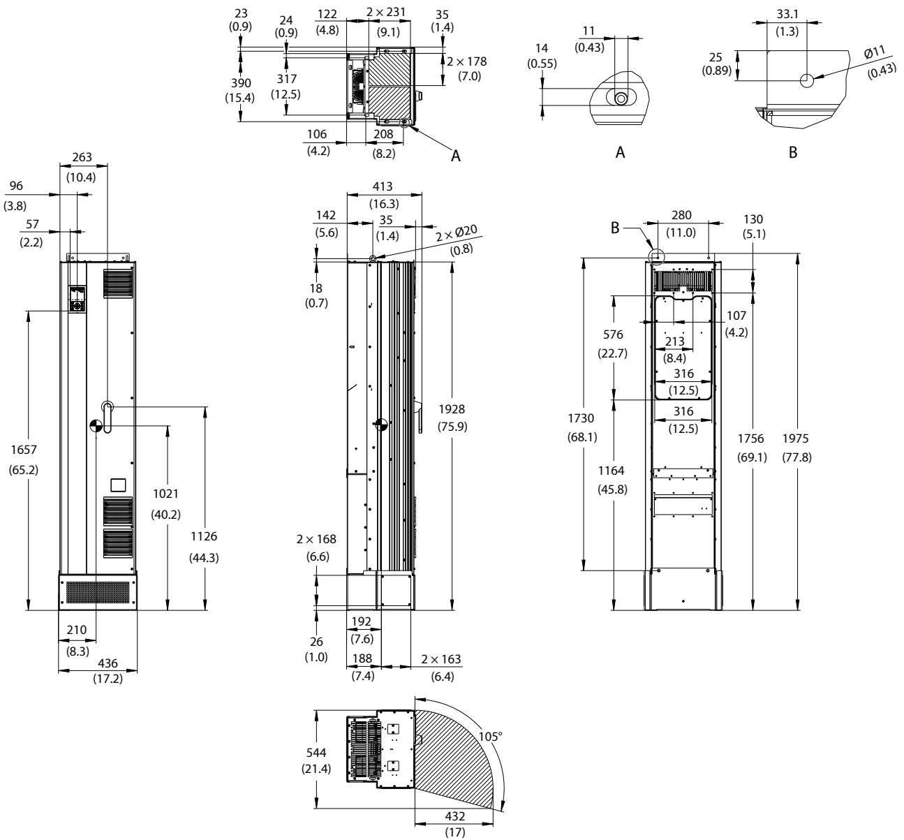
图 40: FK10c 尺寸
