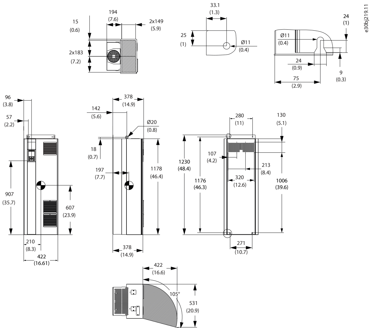
图 38: FK10a 尺寸
