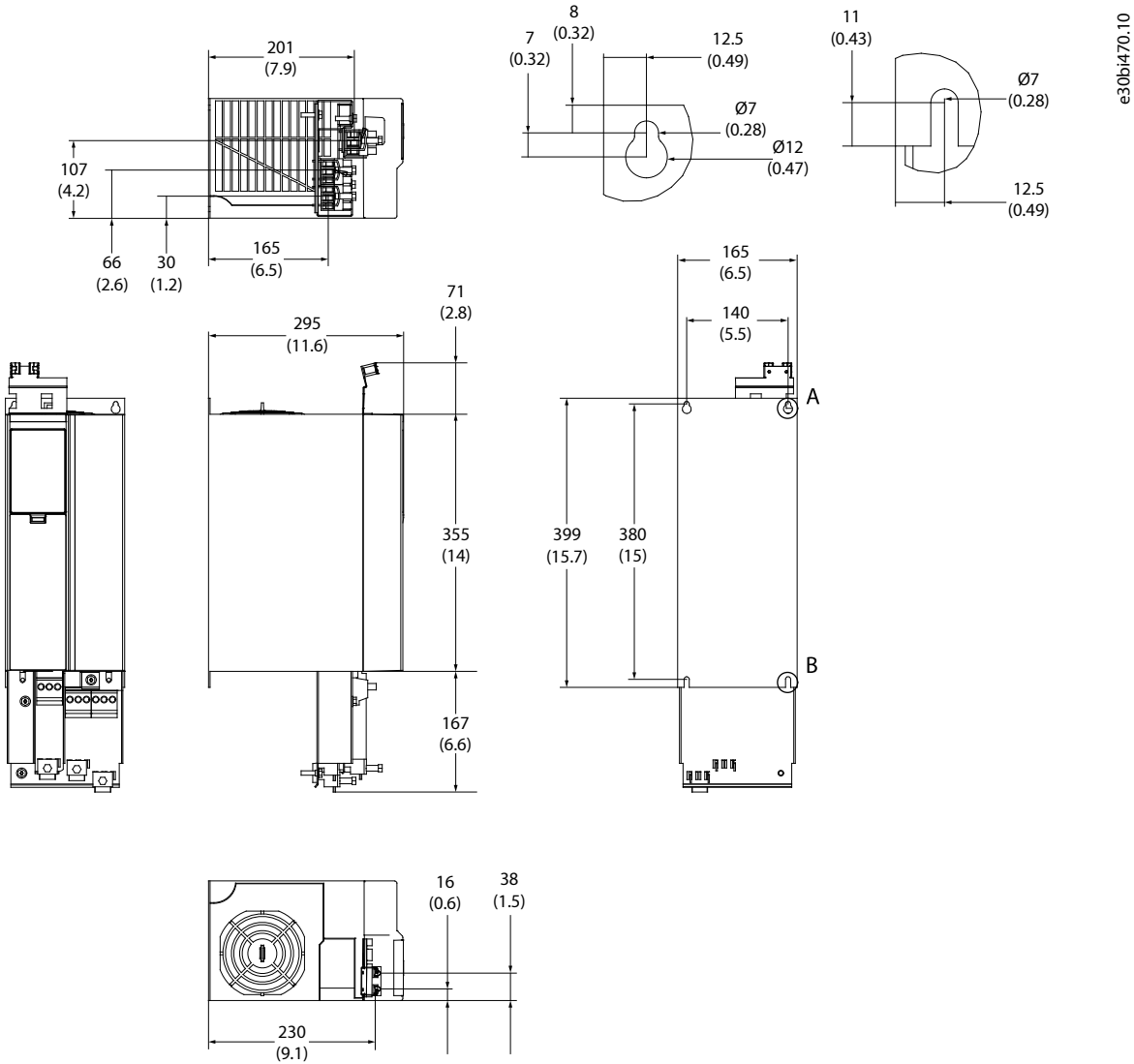
图 19: FA05b 尺寸
