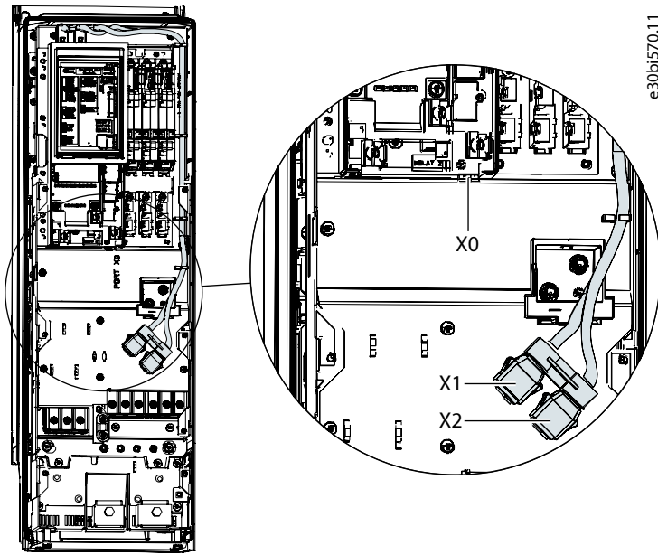
图 88: FK06-FK08 机架中的通信端口 X0、X1 和 X2 位置
