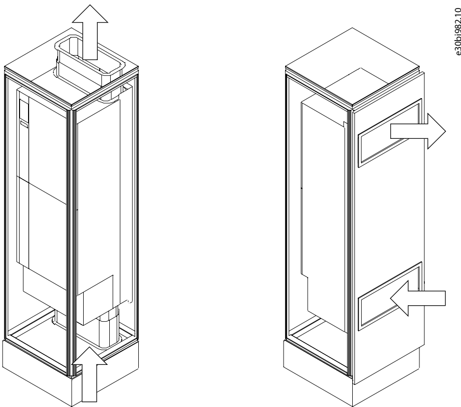
图 77: 背部风道冷却原理示例: 通过风管采用底部进入、顶部排出冷却方式 (左); 通过变频器背面的开口采用背部进入、背部排出冷却方式 (右)
