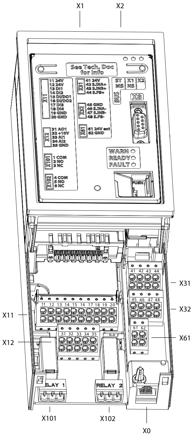
图 84: 不带功能扩展选项的控制板上的连接器位置
