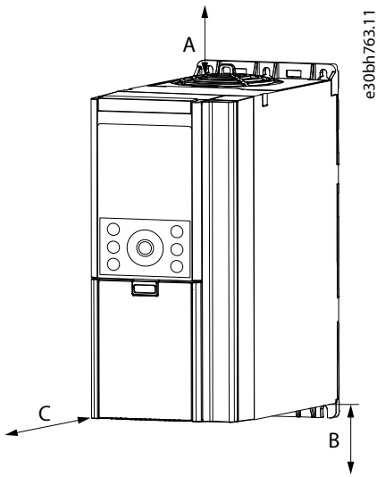
图 78: 建议的维护检修间隙
