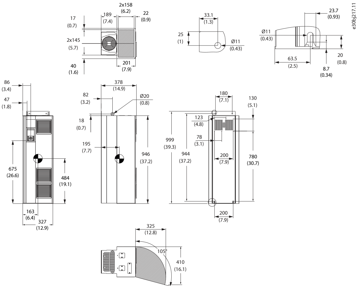
图 34: FK09a 尺寸
