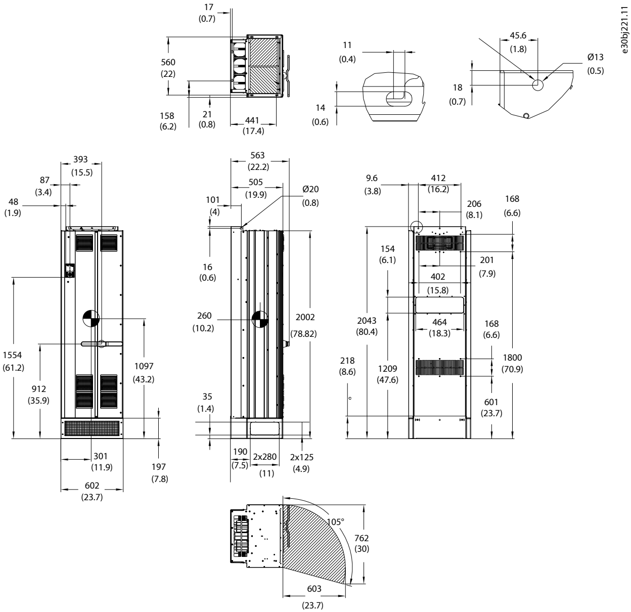
图 41: FK11 尺寸
