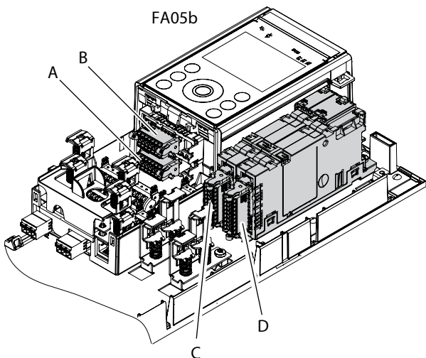
图 7: iC7-Automation 变频器中的选件插槽位置
