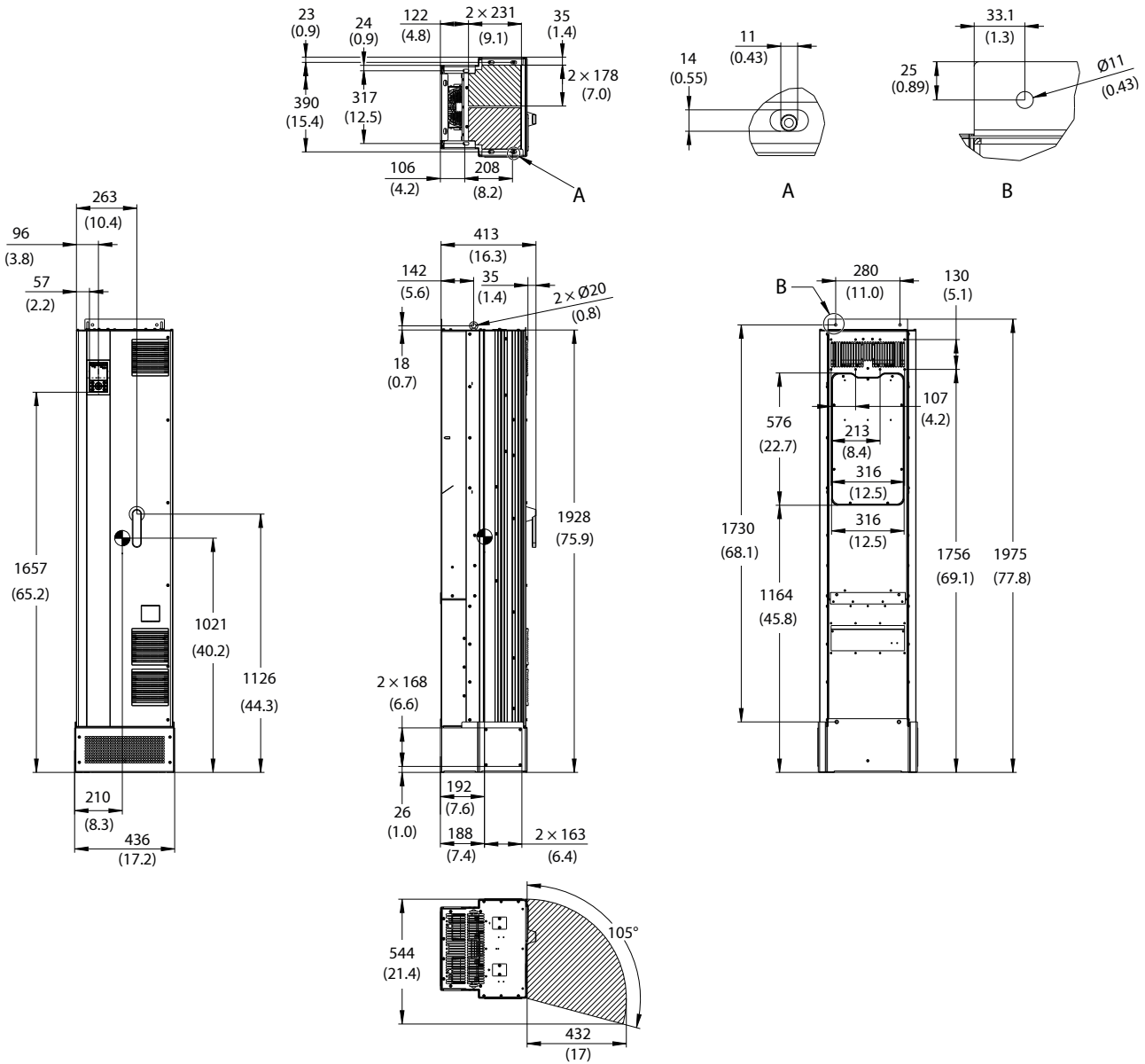
图 49: FB10c 尺寸
