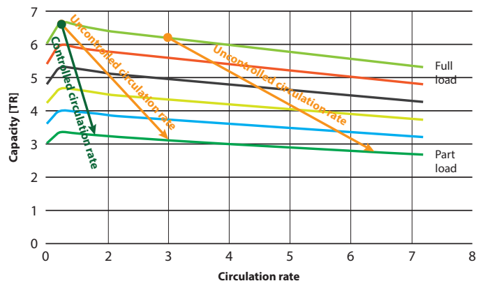
Figure 2: Un système stable NeoCharge alimente chaque évaporateur avec la quantité exacte de réfrigérant en continu. Même lors des charges partielles, le taux de circulation reste fixe. Grâce au contrôle dynamique de NeoCharge, tous les processus de refroidissement restent stables.
