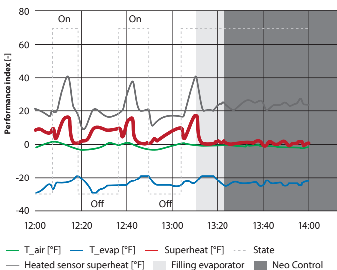
Figures 7 et 8 : Économies d'énergie dans les systèmes à détente directe
