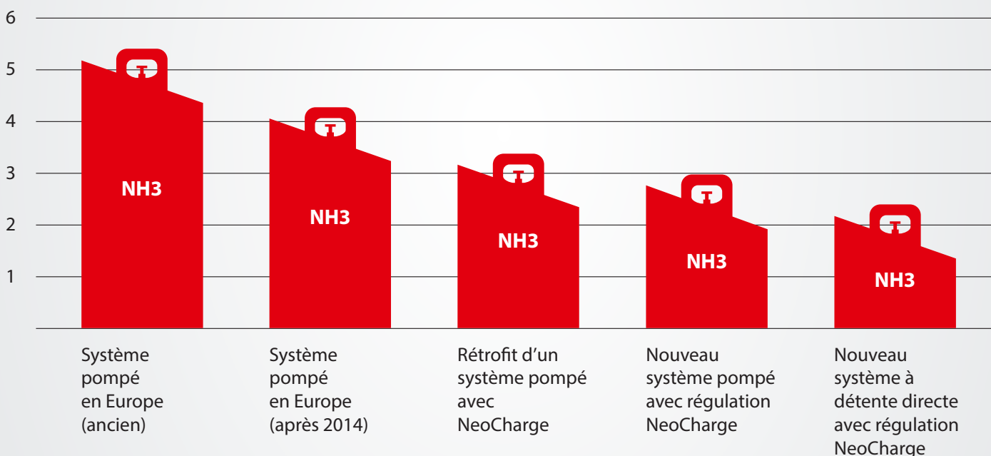
Figure 3 : Réduction de la charge avec NeoCharge
