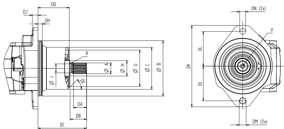
フレームサイズ 060 のシャフト寸法, mm [in]
