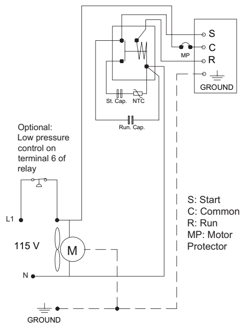
Wiring Diagram 119-9262
