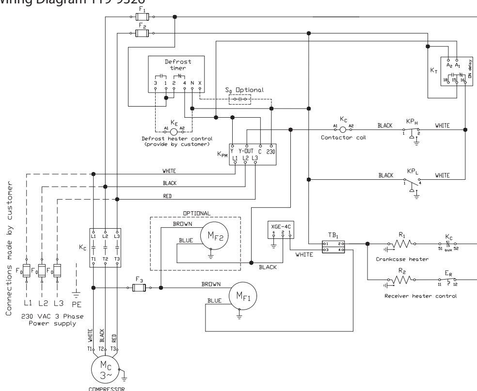
Wiring Diagram 119-9326
