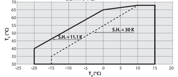
R407C 露点状态 - SZ084-185
