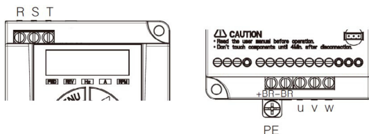
主回路端子示意图
