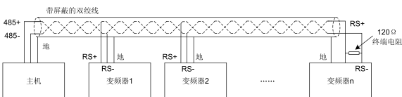
单主机/多从机方式
