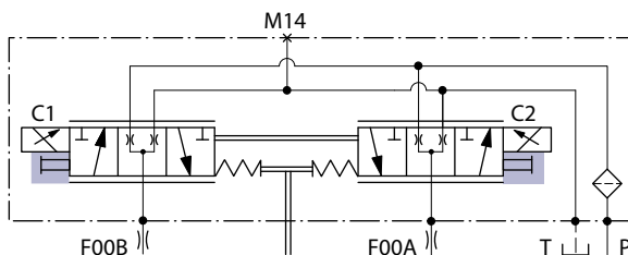
斜板からのフィードバック機構
