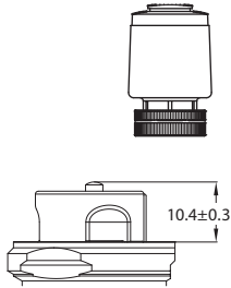
DN 15-32의 폐쇄 지점(기준)
