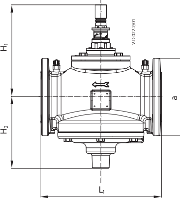
AB-QM DN 50-100
