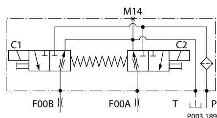
3 ポジション電気コントロール、油圧回路図
