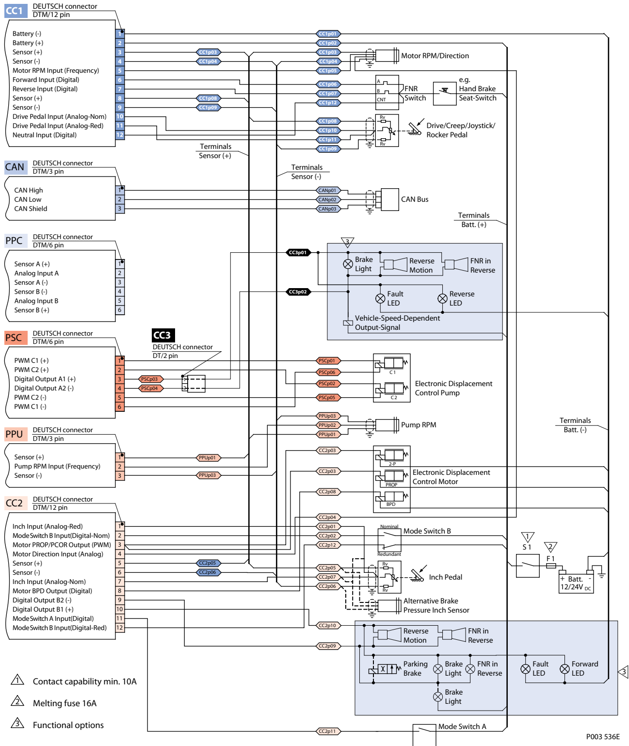
オートモーティブコントロール接続図
