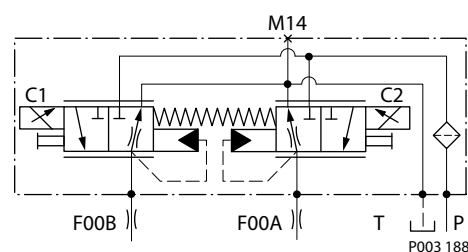
NFPE 回路図
