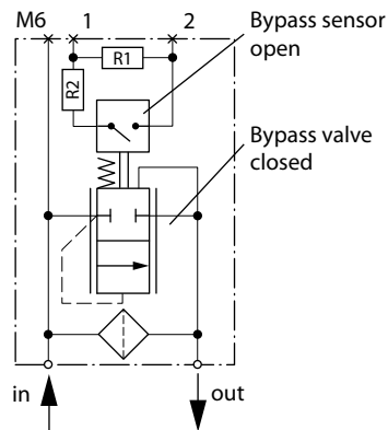
回路図
