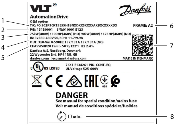
Obrázok 1: Príklad štítka výrobku
