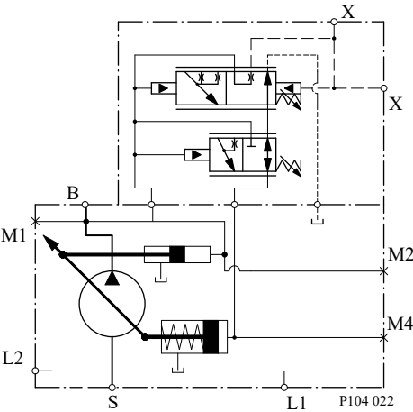
回路図
