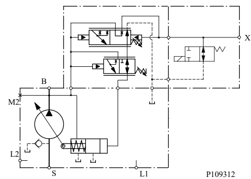
回路図
