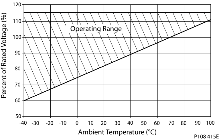
連続作動温度比率
