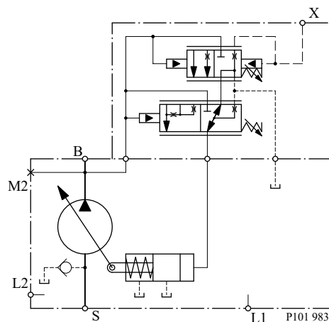
LB 回路図
