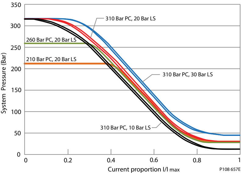
動作圧力と入力電流 (N.C. EPC)
