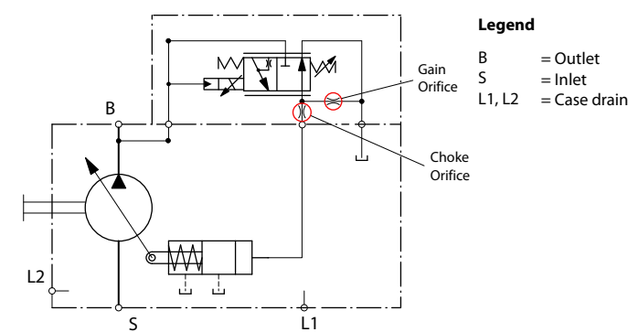
ファン駆動コントロールの回路図
