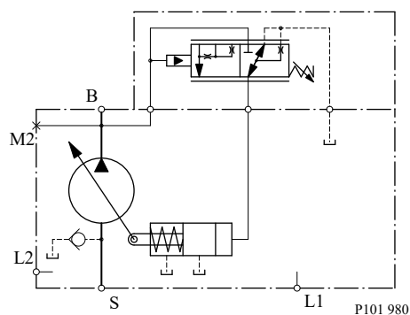
回路図
