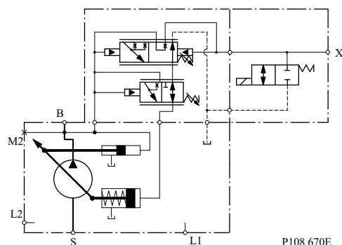
回路図
