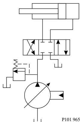
単純なクローズセンター回路
