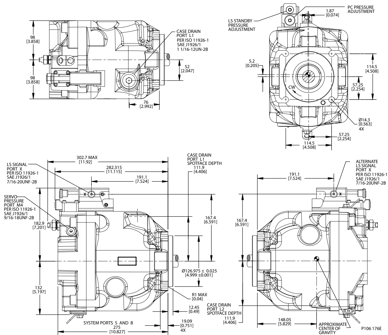
アキシャルポートエンドキャップ寸法
