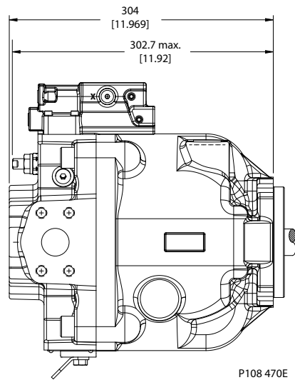
外形寸法
