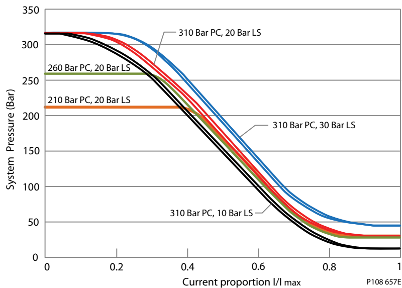
動作圧力と入力電流 (N.C. EPC)
