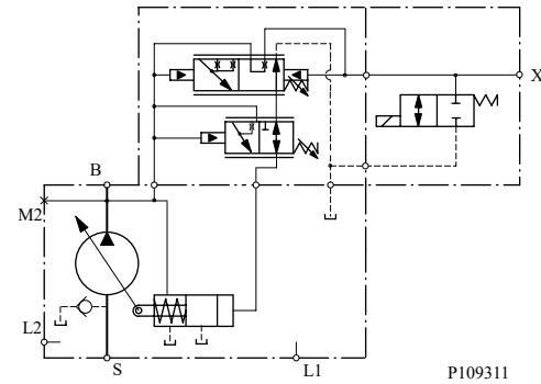
回路図
