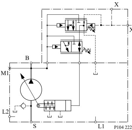
回路図
