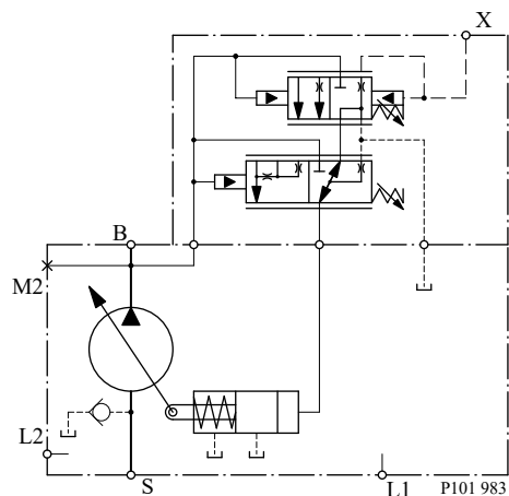
LB 回路図
