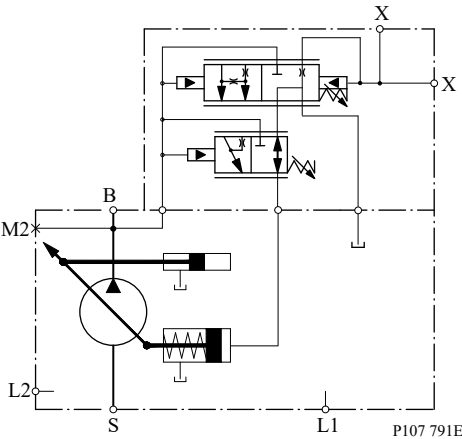
回路図
