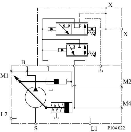
回路図
