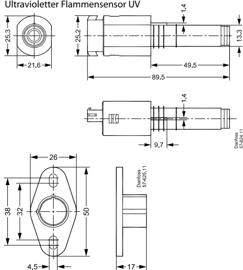
Flansch
