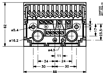
Unterteil 057H7210
