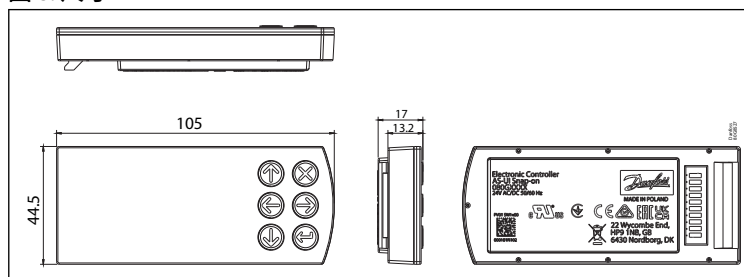
图 10: 尺寸
