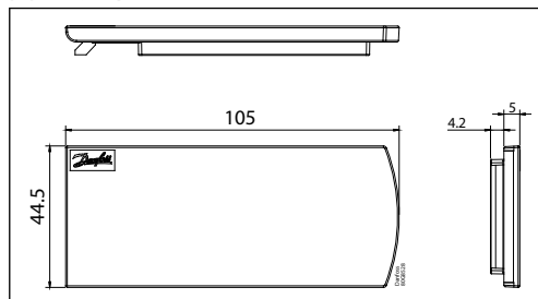
图 10: 尺寸
