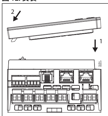
图 12: 安装
