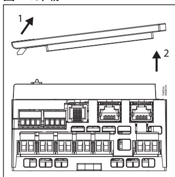
图 11: 卸载
