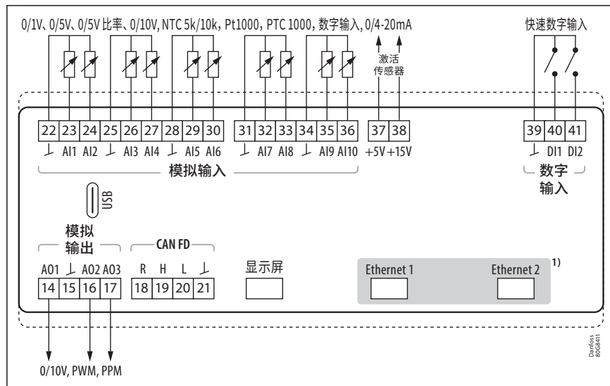
图 3: 顶板
