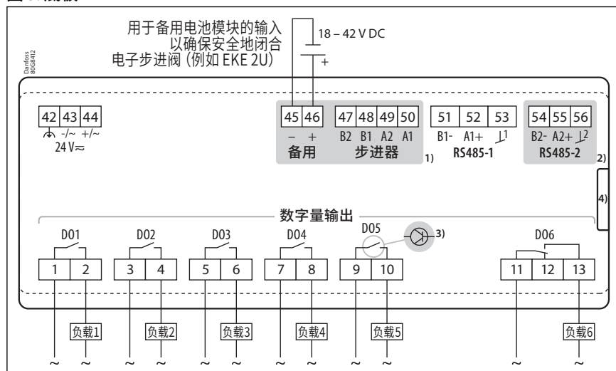
图 5: 底板
