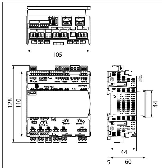
图 1: 不带 LCD 显示屏
