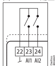
图 4: AI - DI 配置
