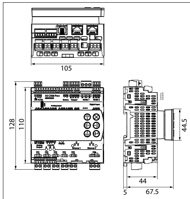
图 2: 带卡扣式 LCD 显示屏 :080G6016
