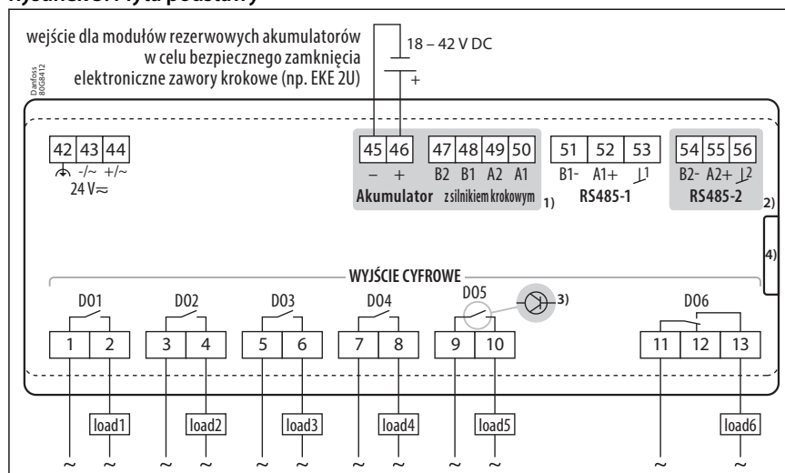
Rysunek 5: Płyta podstawy
