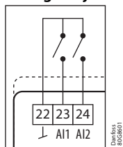
Rysunek 4: AI – Konfiguracja DI
