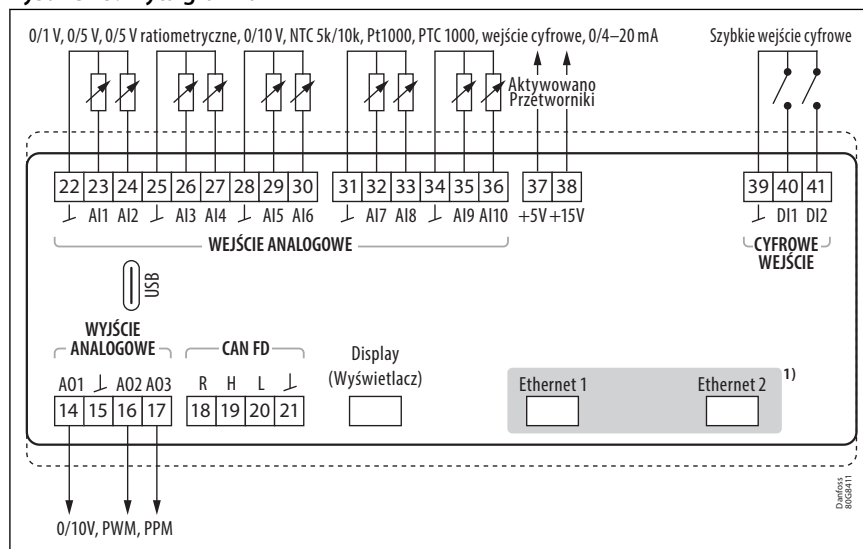
Rysunek 3: Płyta główna
