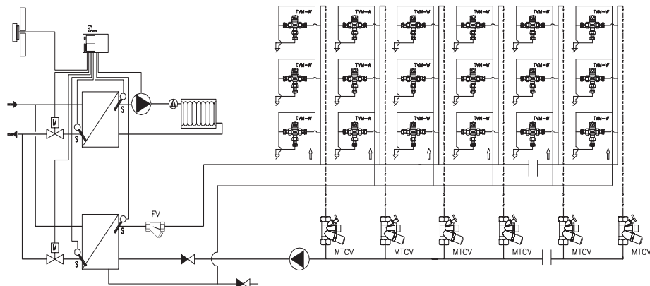
Fig. 8 Schema instalației de apă caldă cu recirculare - versiunea automată.
