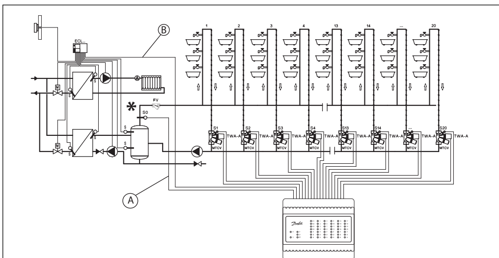
Fig. 11 - schema di installazione per la disinfezione e la registrazione della temperatura
