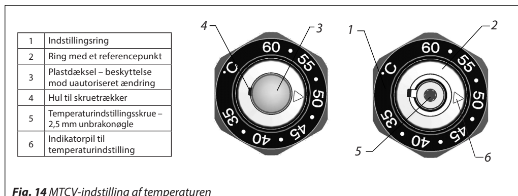
Fig. 14 MTCV-indstilling af temperaturen
