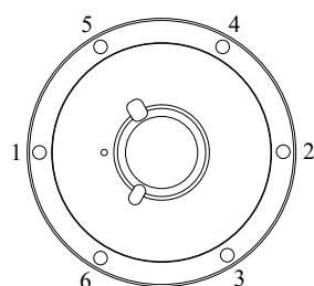
カバー (K550) のトルク順序
