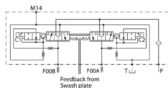
NFPE 回路図
