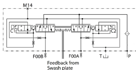
NFPE 回路図
