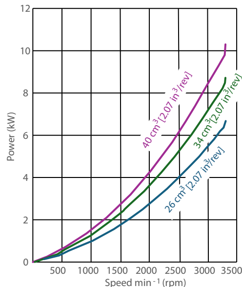
必要チャージポンプ動力
