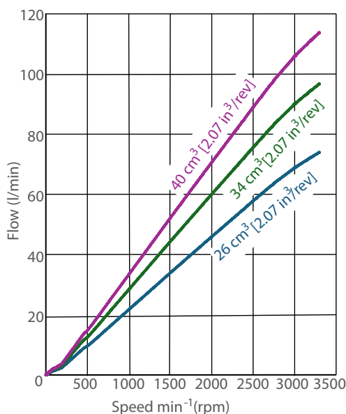
チャージポンプ流量
