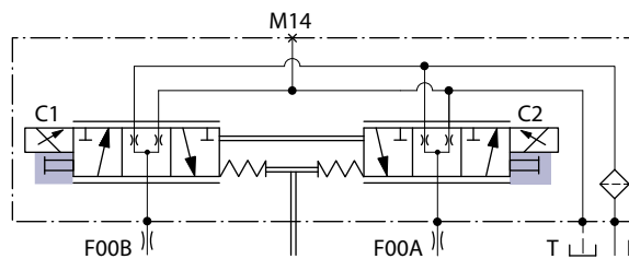
斜板からのフィードバック機構
