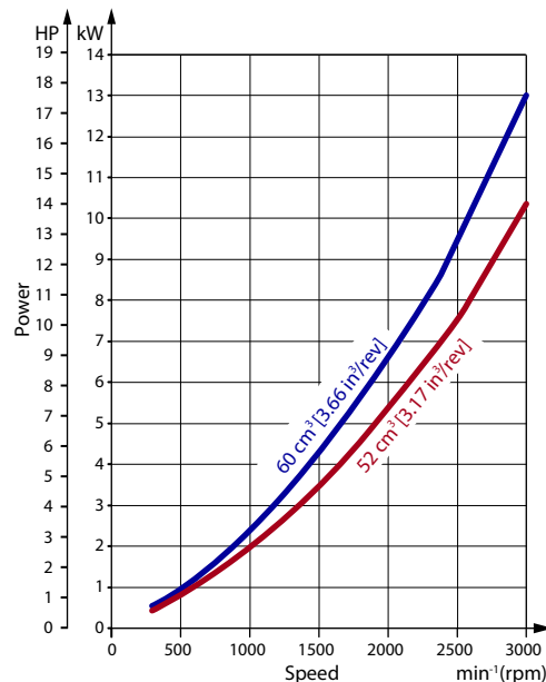
必要チャージポンプ動力
