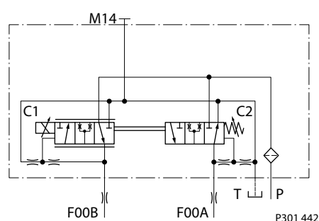
FDC 回路図
