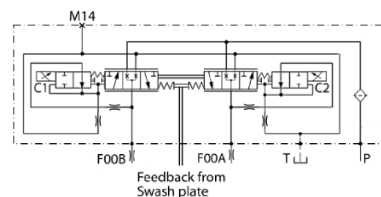
NFPE 回路図
