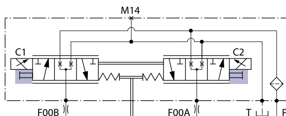
斜板からのフィードバック機構
