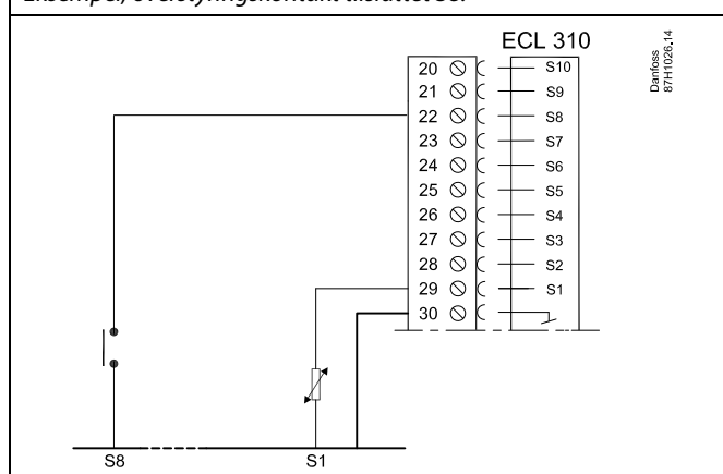
Eksempel, overstyringskontakt tilsluttet S8:
