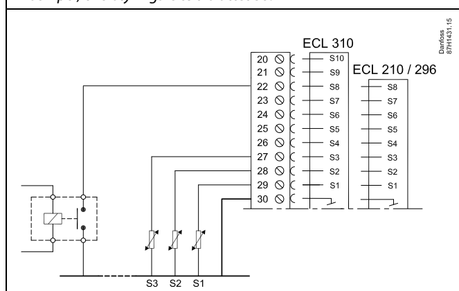
Eksempel, overstyringsrelæ tilsluttet S8:
