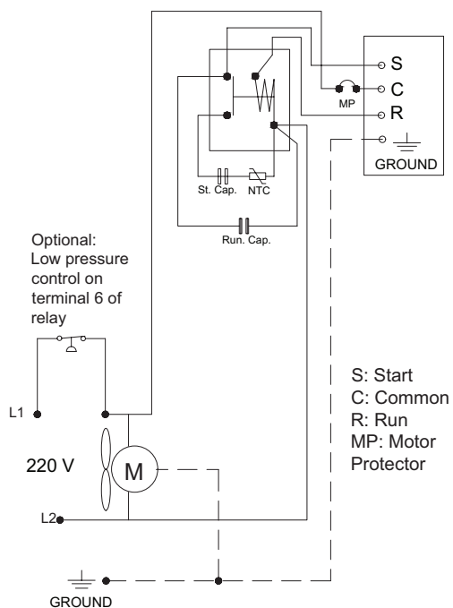
Wiring Diagram 119-9263
