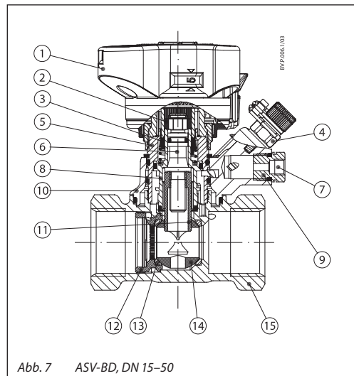
Abb. 7 ASV-BD, DN 15–50
