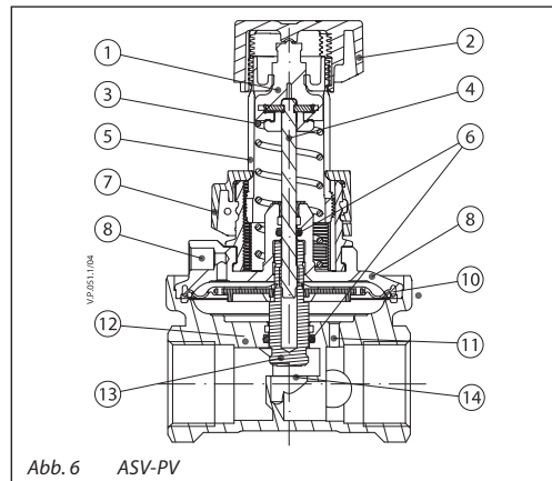
Abb. 6 ASV-PV
