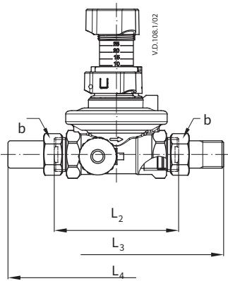
外螺纹 (ISO 228/1)
