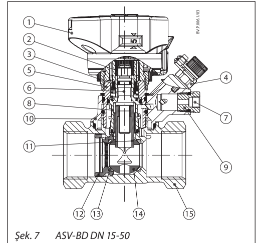
Şek. 7 ASV-BD DN 15-50
