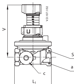
Unutrašnji navoj (ISO 7/1)
