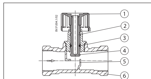
Obr. 8 ASV–M
