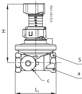
Vnitřní závit (ISO 7/1)
