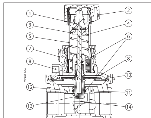
Obr. 6 ASV–PV
