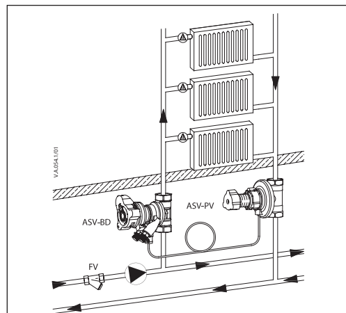
Fig. 3 Solución ASV en columna/aplicación típica de calefacción con radiadores (ejemplo general)
