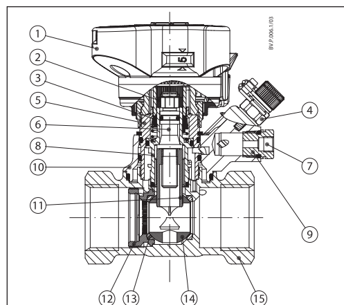
7. ábra ASV-BD DN 15–50
