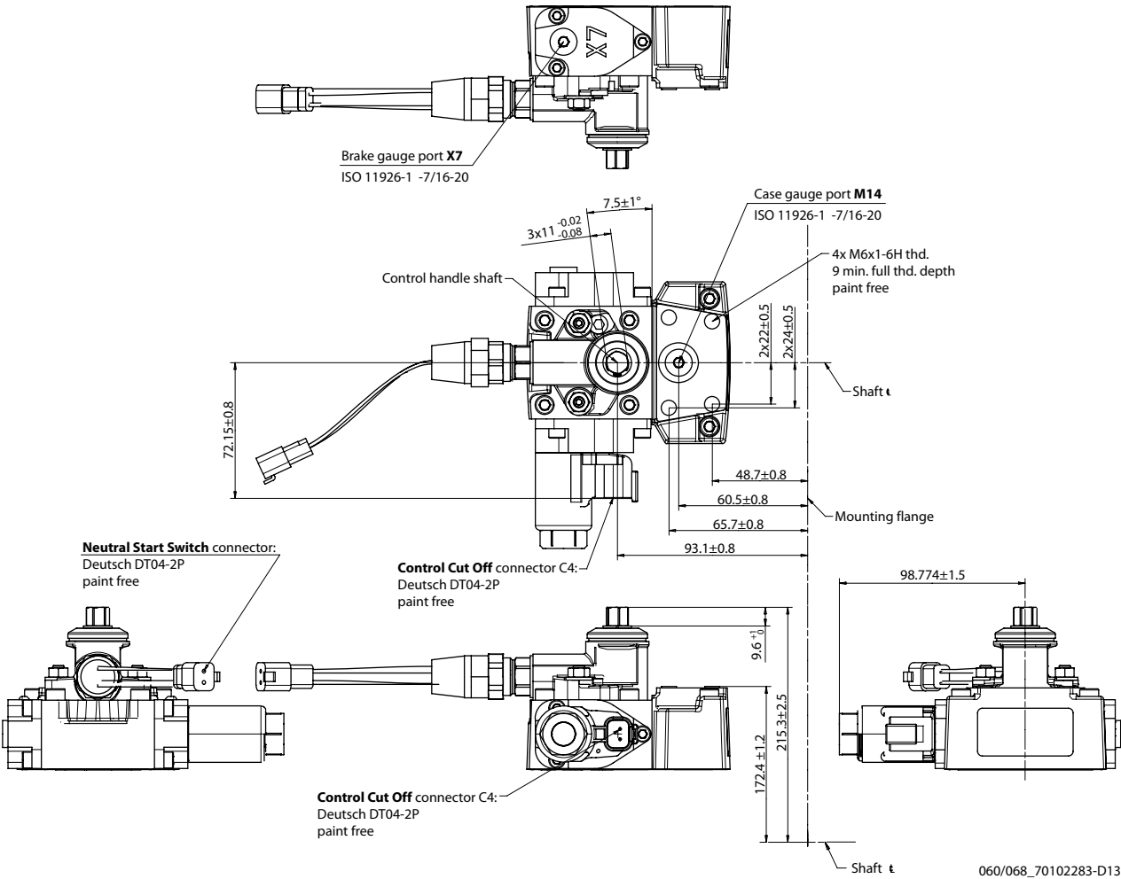
Connector DEUTSCH, 2-pin
