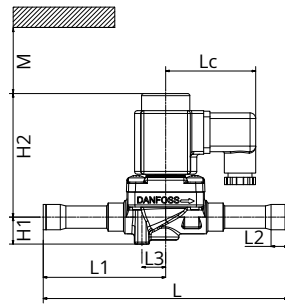
Figure: EVR and DIN plug coil
