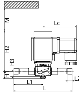
Figure: EVRC and DIN plug coil
