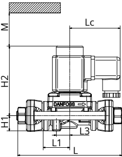
Figure: EVR and DIN plug coil
