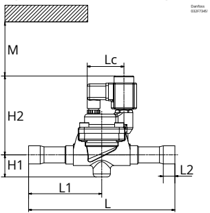
Figure: EVR and DIN plug coil
