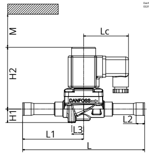
Figure: EVR and DIN plug coil
