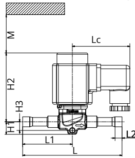
Figure: EVR and DIN plug coil
