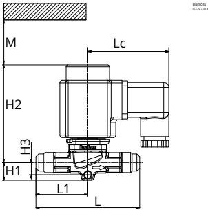
Figure: EVR and DIN plug coil
