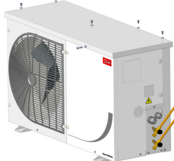
Krok 2: Odkręcić wszystkie śruby panelu górnego, a następnie zdjąć go.
