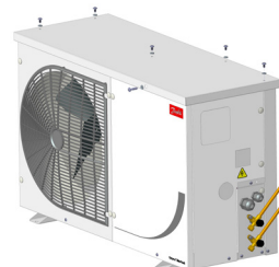
Passo 2: Retire todos os parafusos do painel superior e, em seguida, retire o painel superior.
