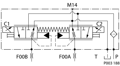
NFPE 回路図
