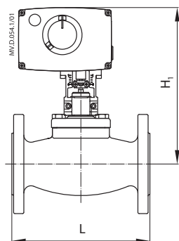
VFS 2 + AMV(E) 25, 35
