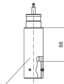
Подовжувач штоку 065Z7548 для VFS2 (DN15...50мм) при температурі більше 150 °C
