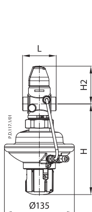
AVPQ DN 15-50 \Delta p_s = 0,2-1,0 бар
