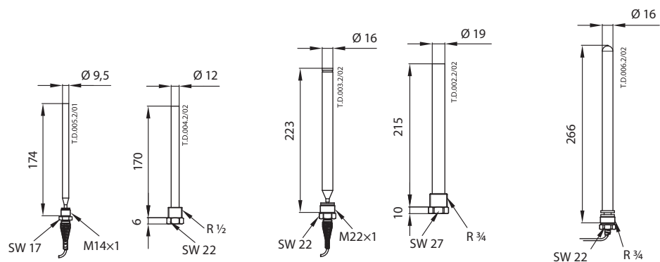
AVT 170 mm
