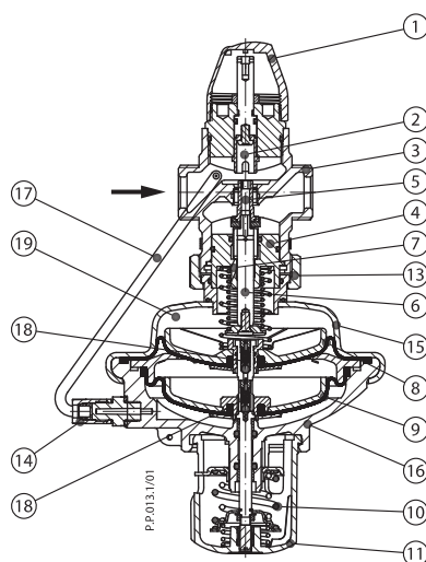
AVPQ (0,2-1,0 бар)
