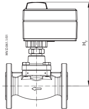
VB2 + AMV(E) 10
