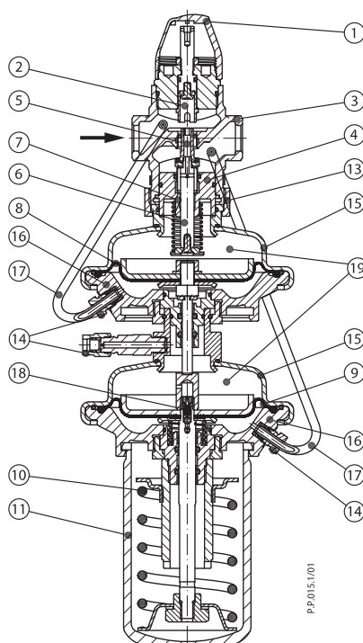
AVPQ4
