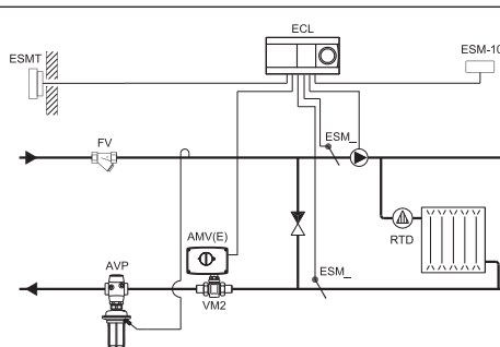
Залежна система опалення
