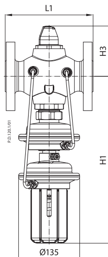
AVPQ 4
