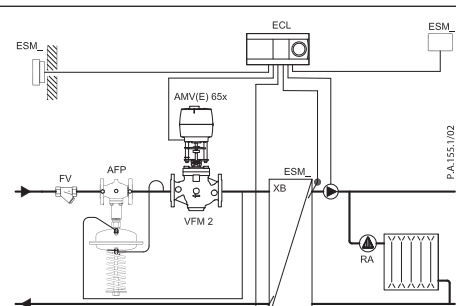
Незалежна система опалення
