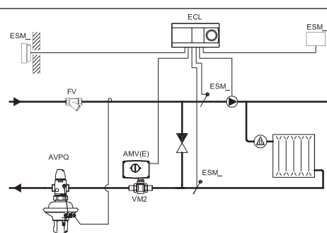
Залежна система опалення
