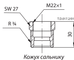
Кожух сальнику
