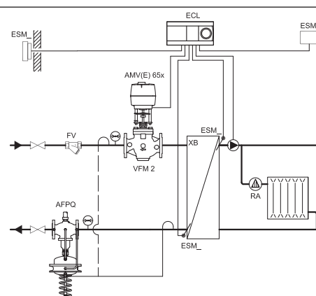
Незалежна система опалення
