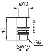
Компресійний фітинг
