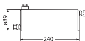
Охолоджувач імпульсу V1
