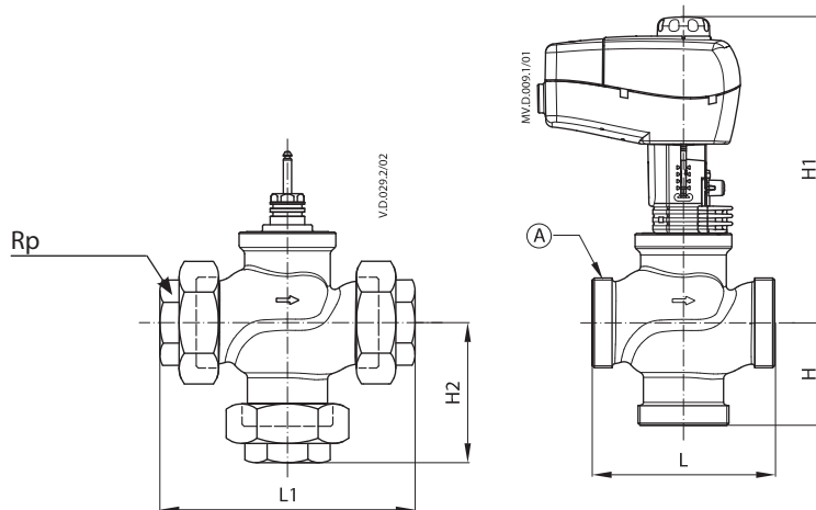
VRG3
