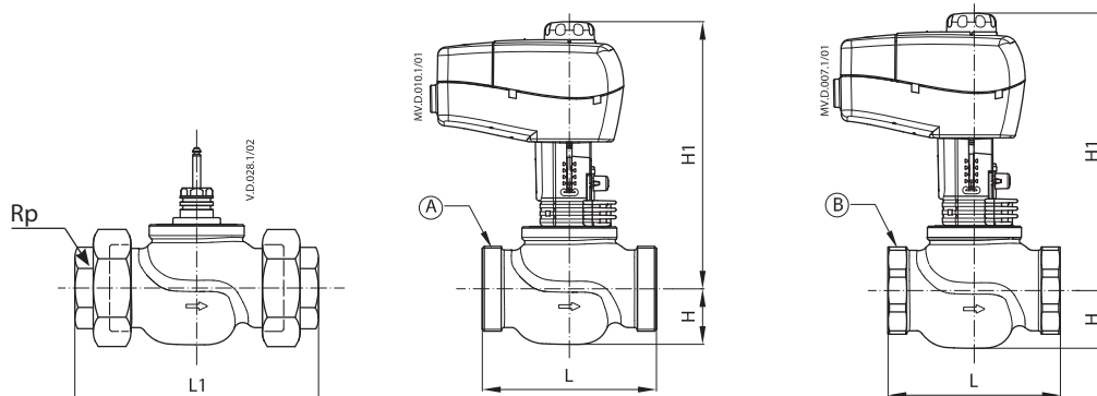
VRB2
