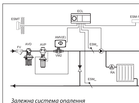
Залежна система опалення
