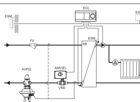
Незалежна система опалення
