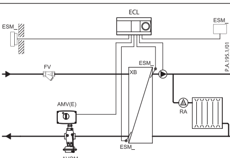
Незалежна система опалення
