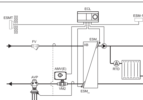
Незалежна система опалення
