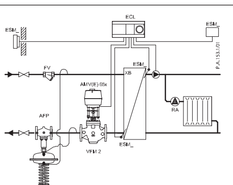
Незалежна система опалення
