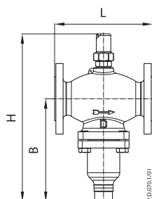
VFQ2, DN 15-125
