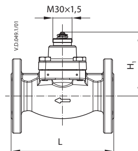
VB2 + AMV(E) 13
