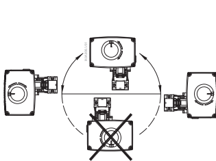
AMV(E) 25(SU/SD)/35
