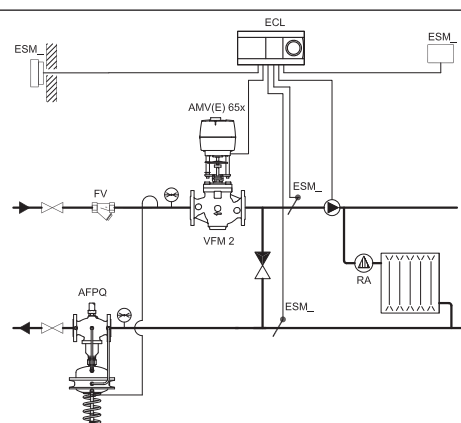
Залежна система опалення
