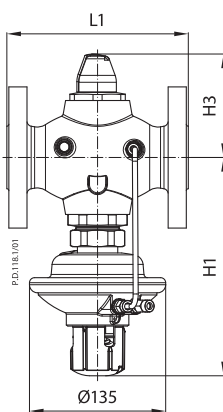
AVPQ DN 32-50 \Delta p_s = 0,2-1,0 бар
