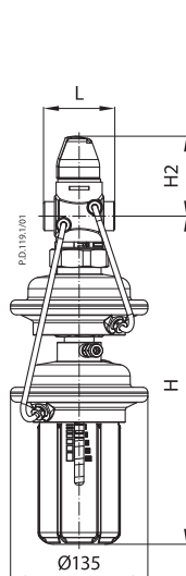
AVPQ 4
