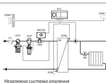
Незалежна система опалення
