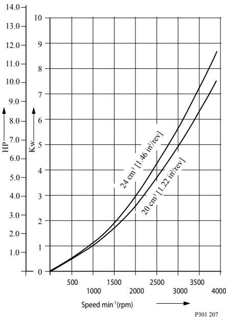
补油泵功率要求
