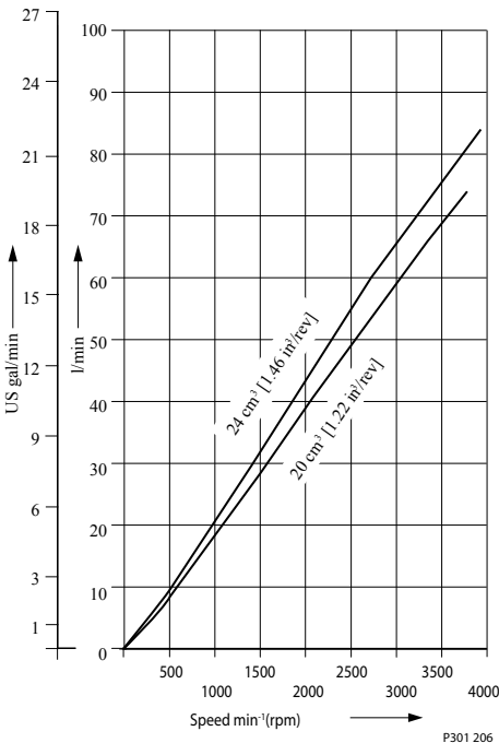
补油泵流量
