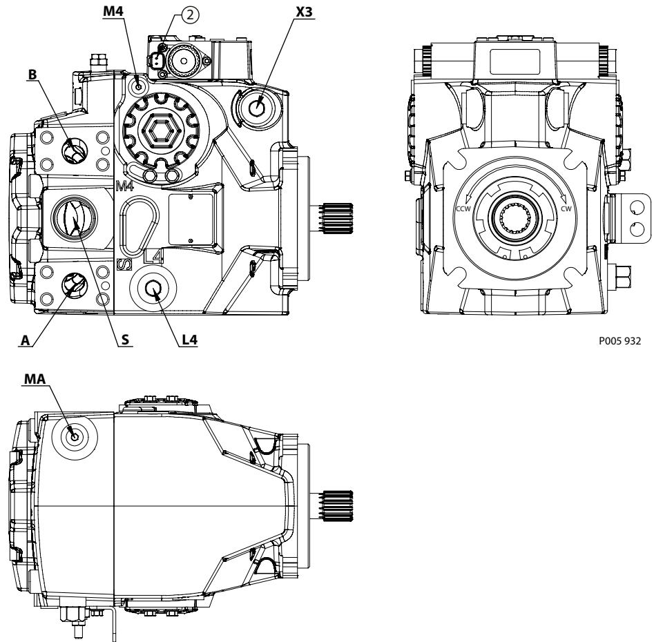
符合 ISO 11926-1 的油口描述
