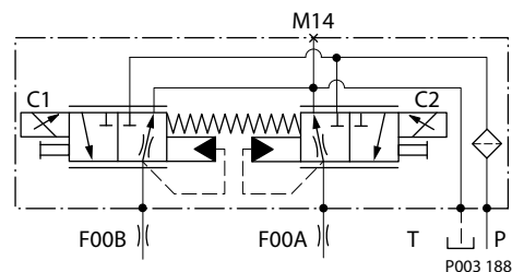
NFPE 原理图
