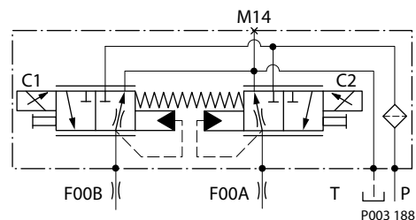
NFPE 原理图
