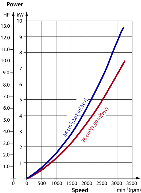
补油泵功率要求
