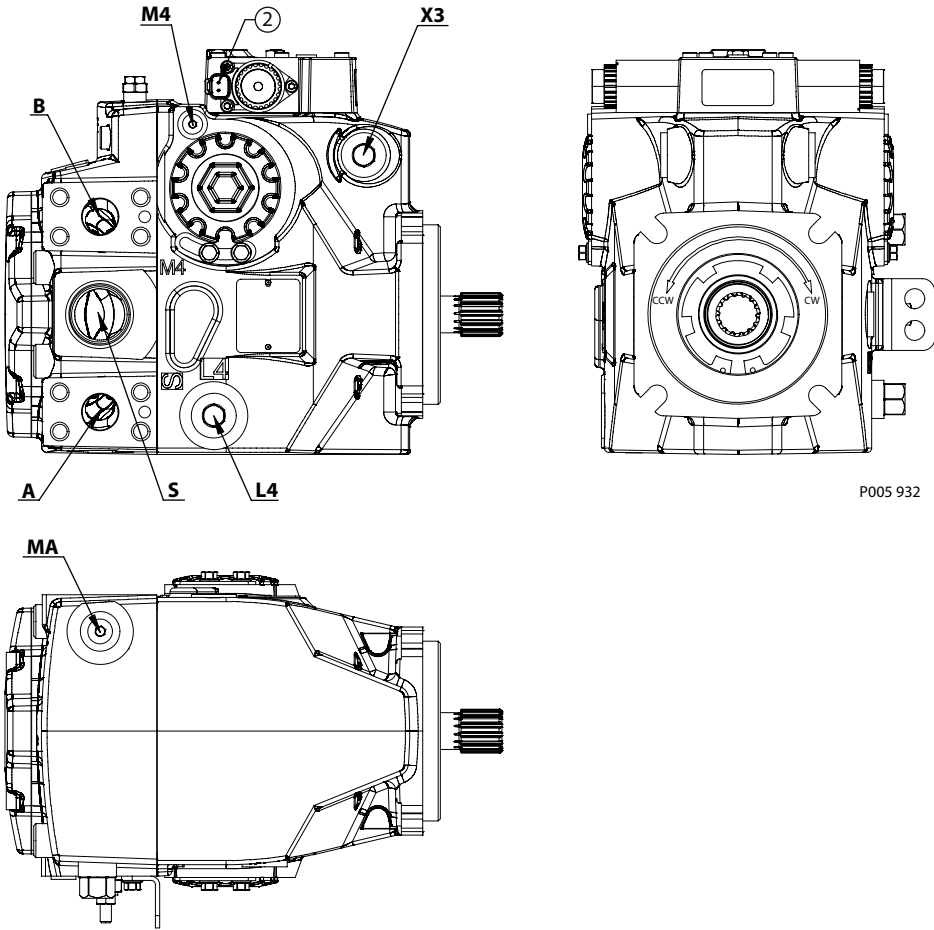
符合 ISO 11926-1 的油口描述
