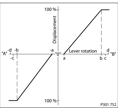
泵排量 vs. 控制手柄转角
