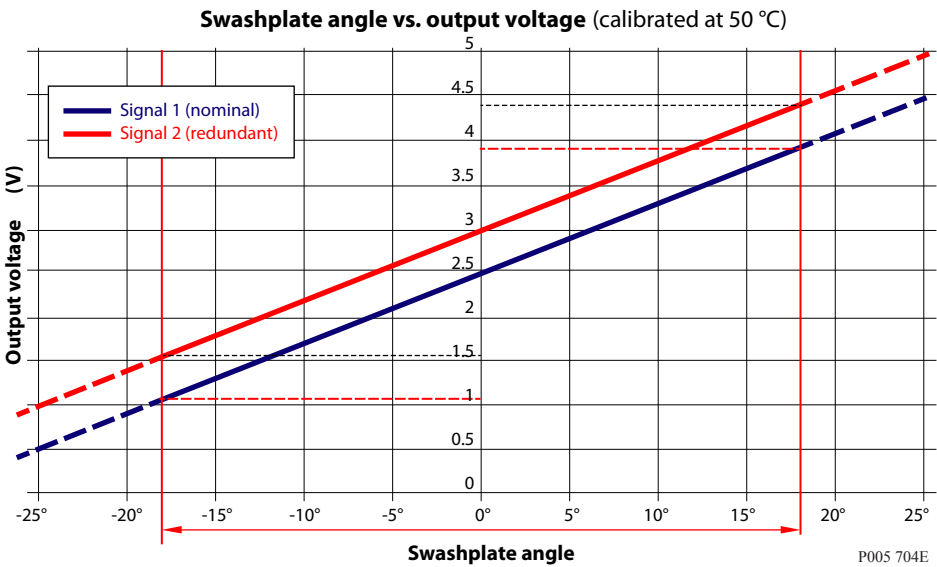
斜盘角度与输出电压
