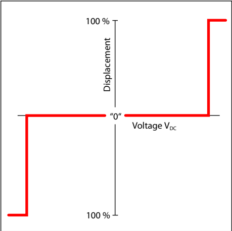
泵排量与电气信号
