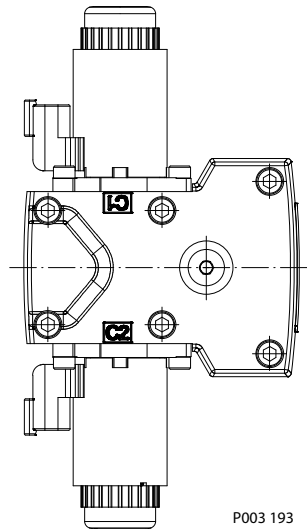
三位电控 (FNR)
