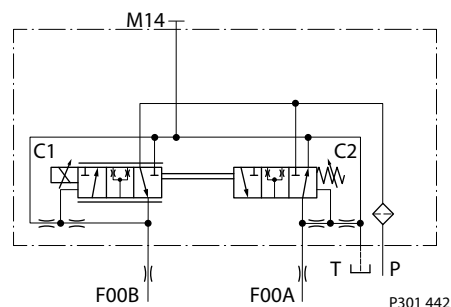
FDC 原理图
