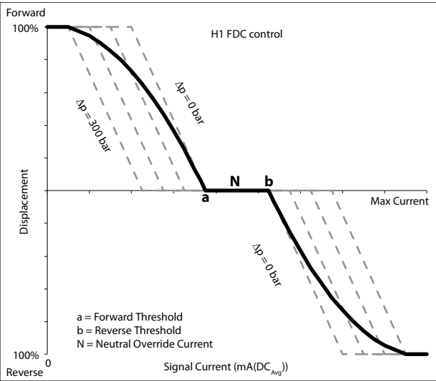
泵排量 vs. 控制电流
