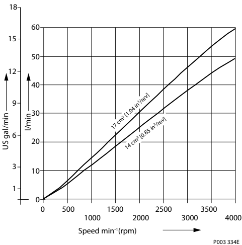
补油泵流量
