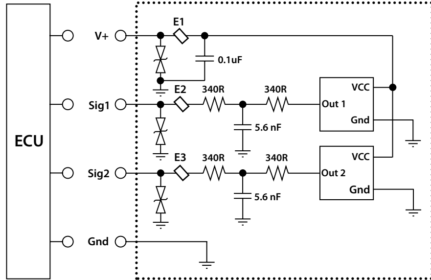
ECU 接口图
