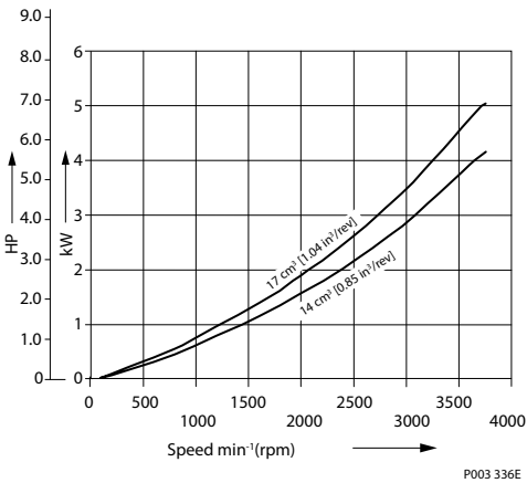
补油泵功率要求
